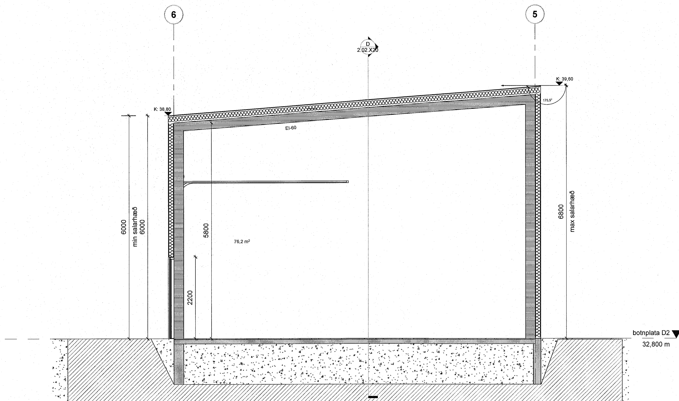
Sneiðing C - byggingar B 1:50
