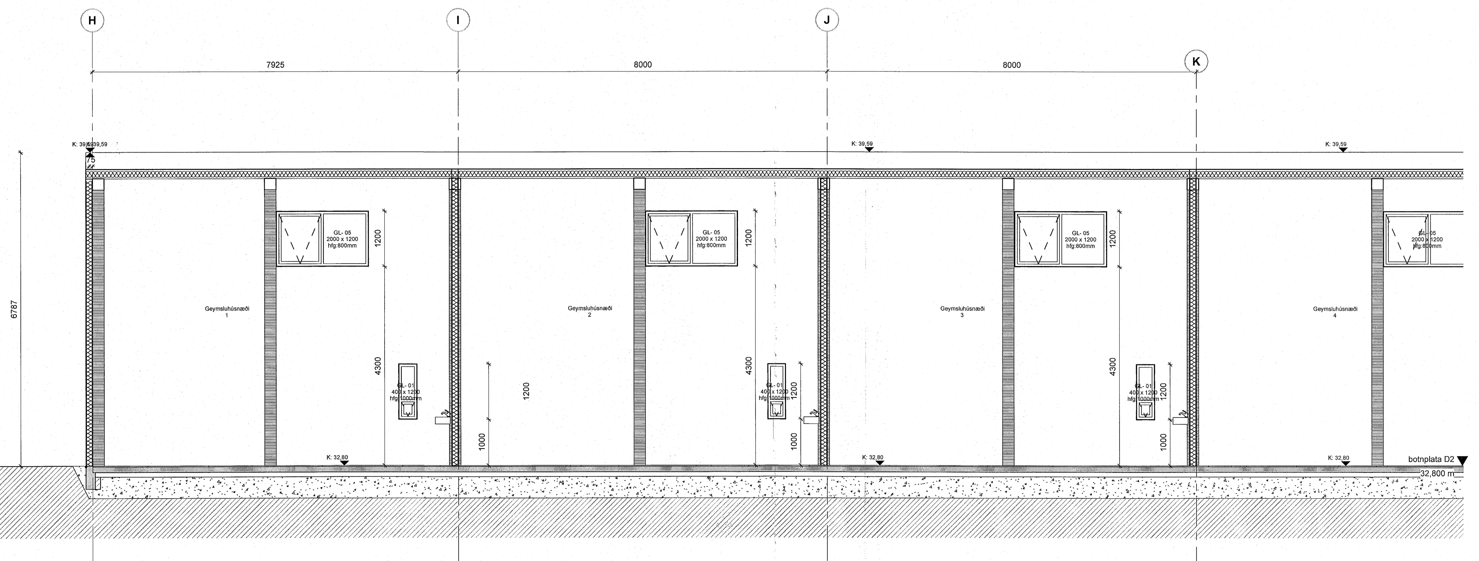
Sneiðing D - bygging B - hluti 1 1:50
