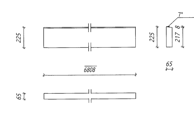
Nr. 111 VR Veggreim Límré: 65*225, L=6808 mm Samtals: 4 stk.
