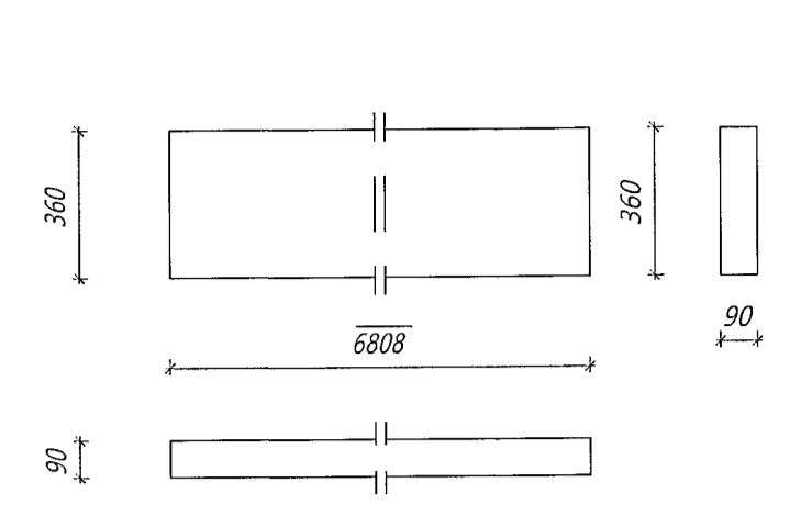
Nr. 106 LB Langband Límré: 90*360, L=6808 mm Samtals: 10 stk.
