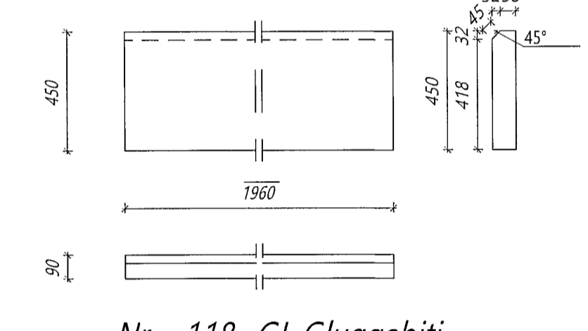
Nr. 118 GL Gluggabiti Límré: 90*450, L=1960 mm Samtals: 28 stk.
