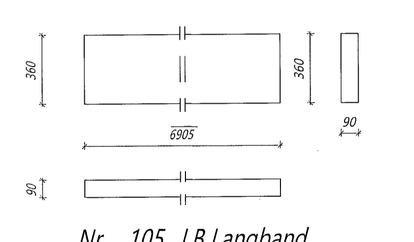
Nr. 105 LB Langband Límré: 90*360, L=6905 mm Samtals: 10 stk.
