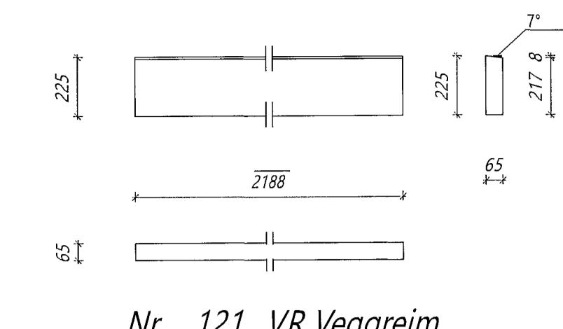
Nr. 121 VR Veggreim Límré: 65*225, L=2188 mm Samtals: 2 stk.
