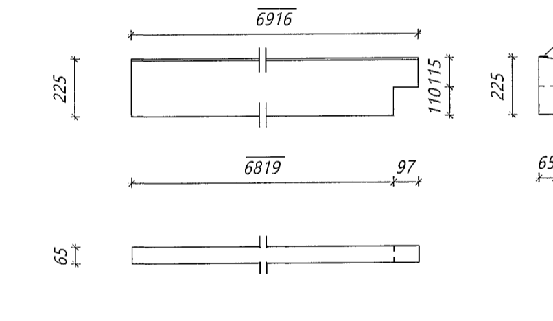
Nr. 114 VR Veggreim Límré: 65*225, L=6916 mm Samtals: 3 stk.
