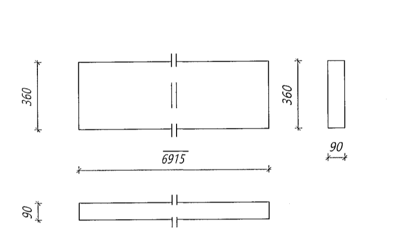
Nr. 103 LB Langband Límré: 90*360, L=6915 mm Samtals: 30 stk.
