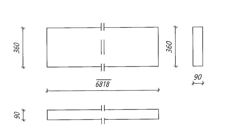
Nr. 104 LB Langband Límré: 90*360, L=6818 mm Samtals: 20 stk.
