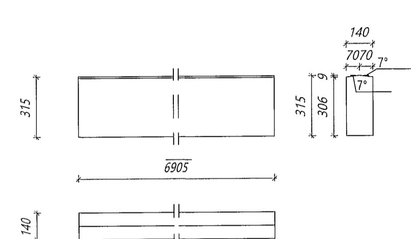
Nr. 102 MB Mænisbiti Límré: 140*315, L=6905 mm Samtals: 1 stk.
