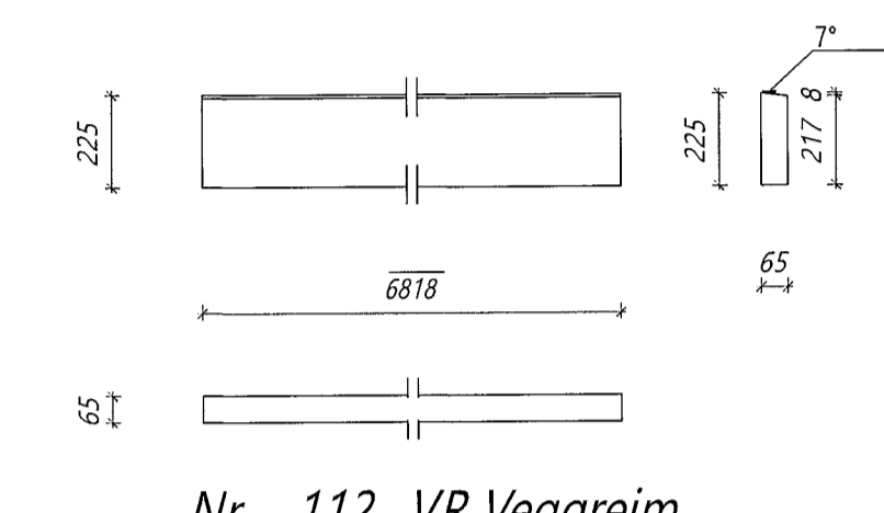
Nr. 112 VR Veggreim Límré: 65*225, L=6818 mm Samtals: 8 stk.
