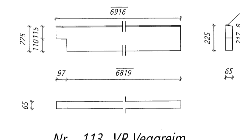
Nr. 113 VR Veggreim Límré: 65*225, L=6916 mm Samtals: 3 stk.
