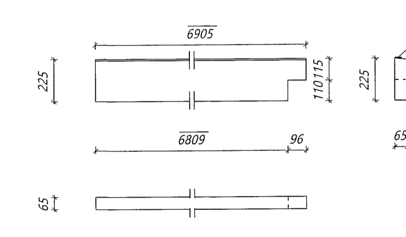
Nr. 115 VR Veggreim Límré: 65*225, L=6906 mm Samtals: 1 stk.
