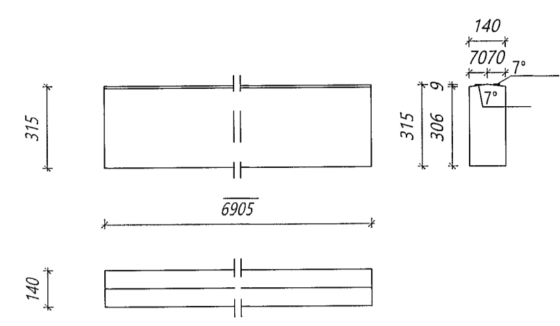
Nr. 101 MB Mænisbiti Límré: 140*315, L=6905 mm Samtals: 1 stk.
