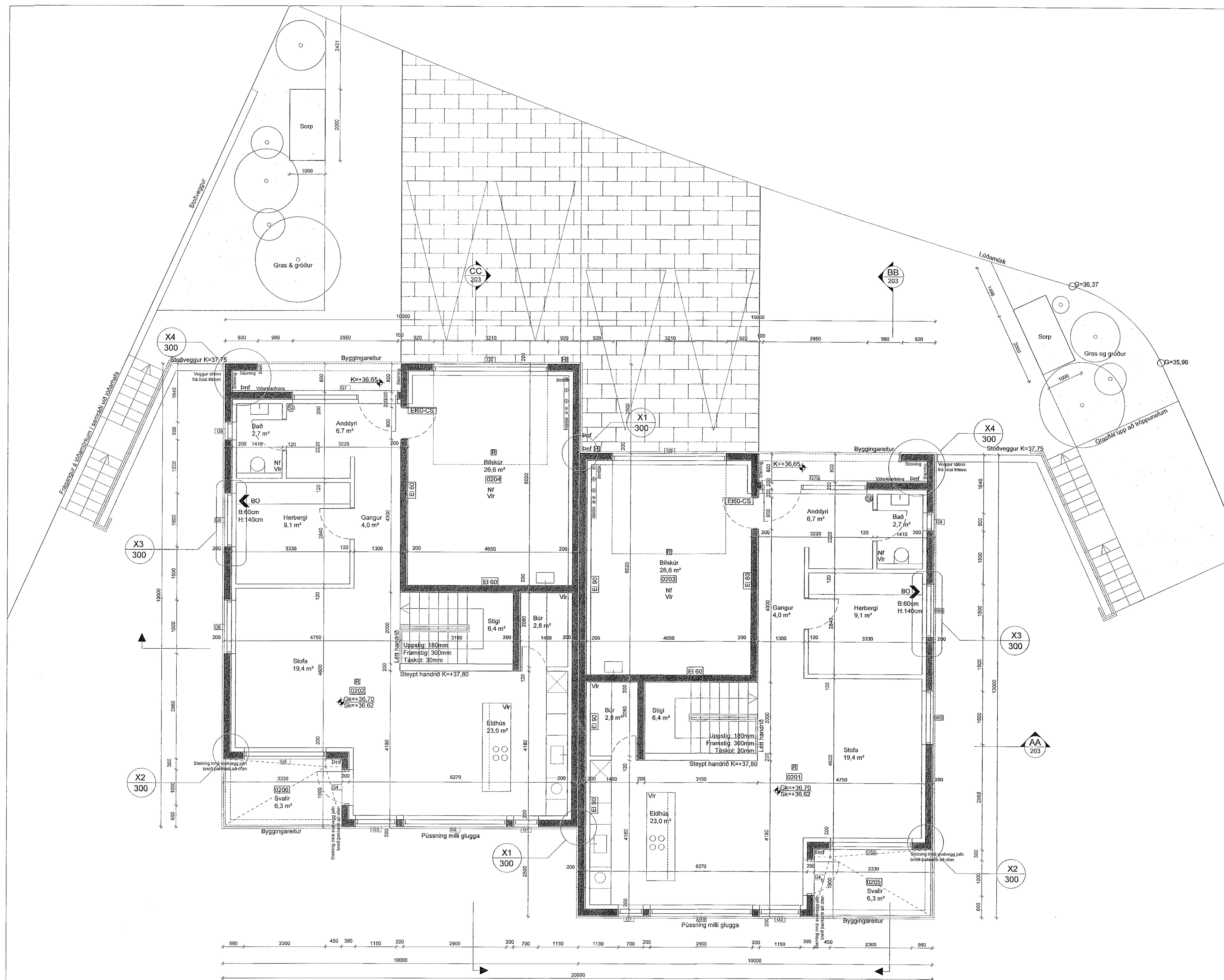
GRUNNMÝND 2.HÆÐ 1:50
