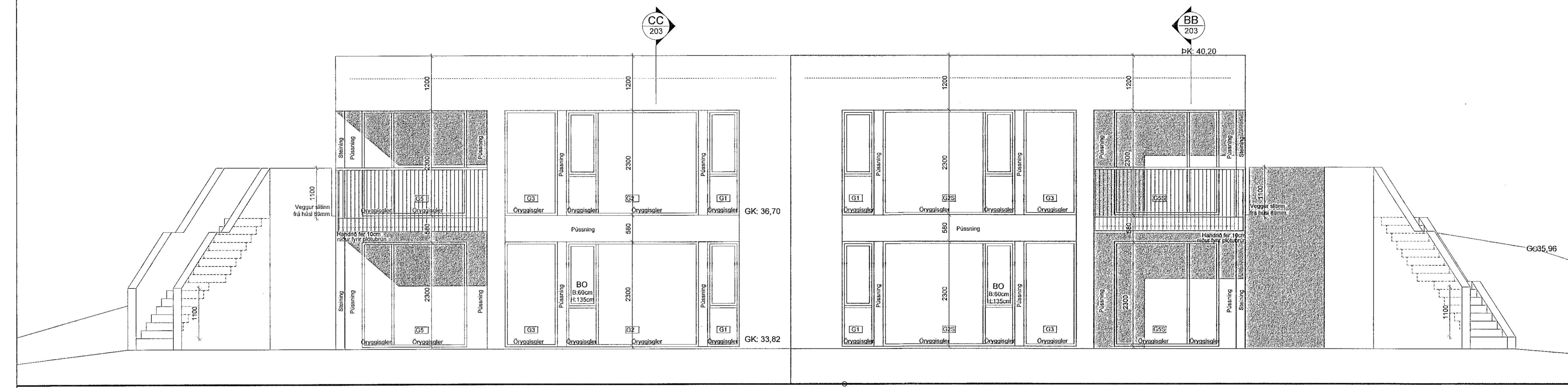
ÚTLIT SUÐ-AUSTUR 1:50
