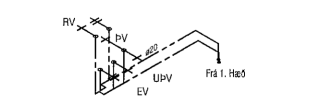
RÚMMYND ÞRÍFALAGNA RAÐHÚS 2. HÆÐ
