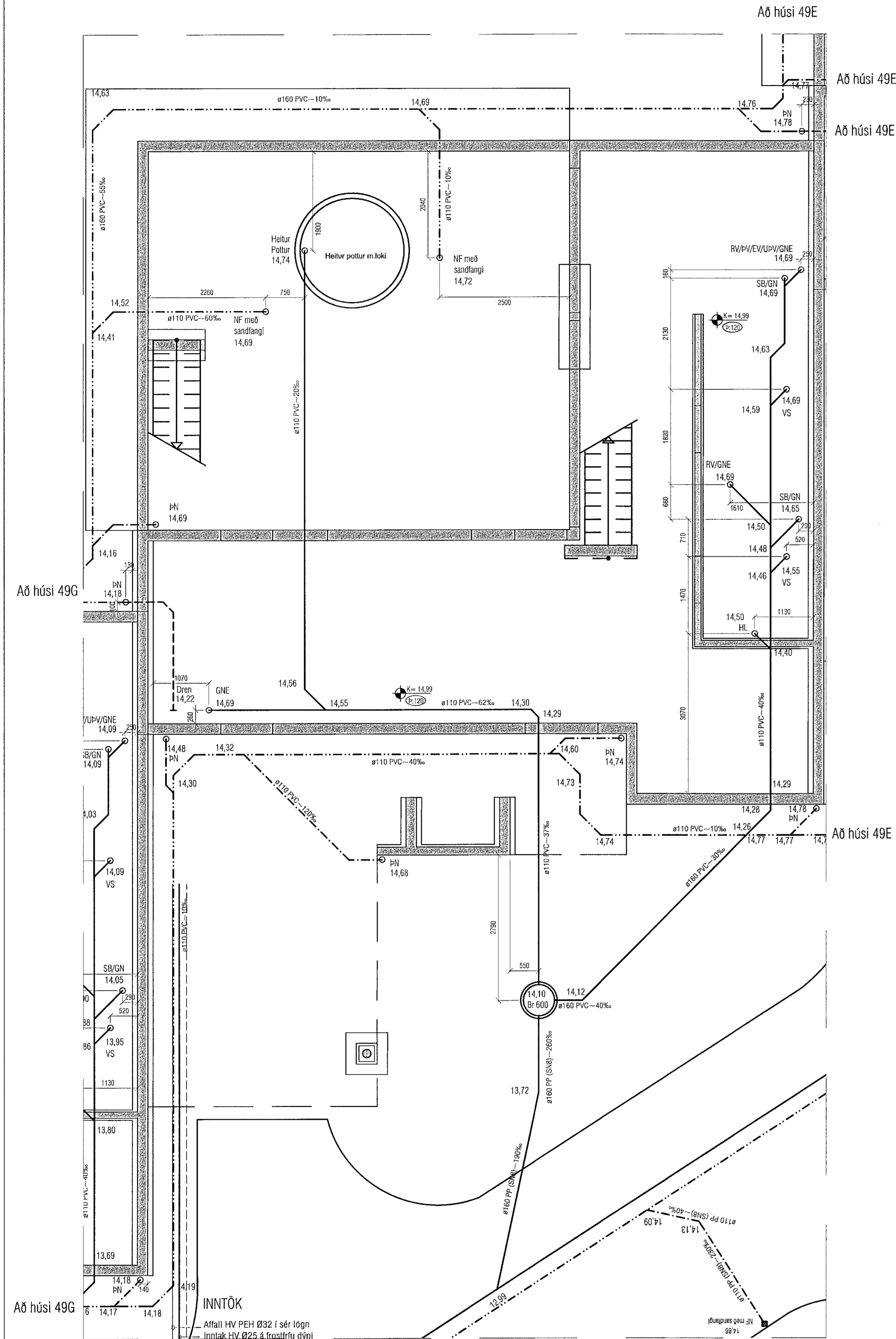
GRUNNMYND JARDLAGNA HÚS 49F
