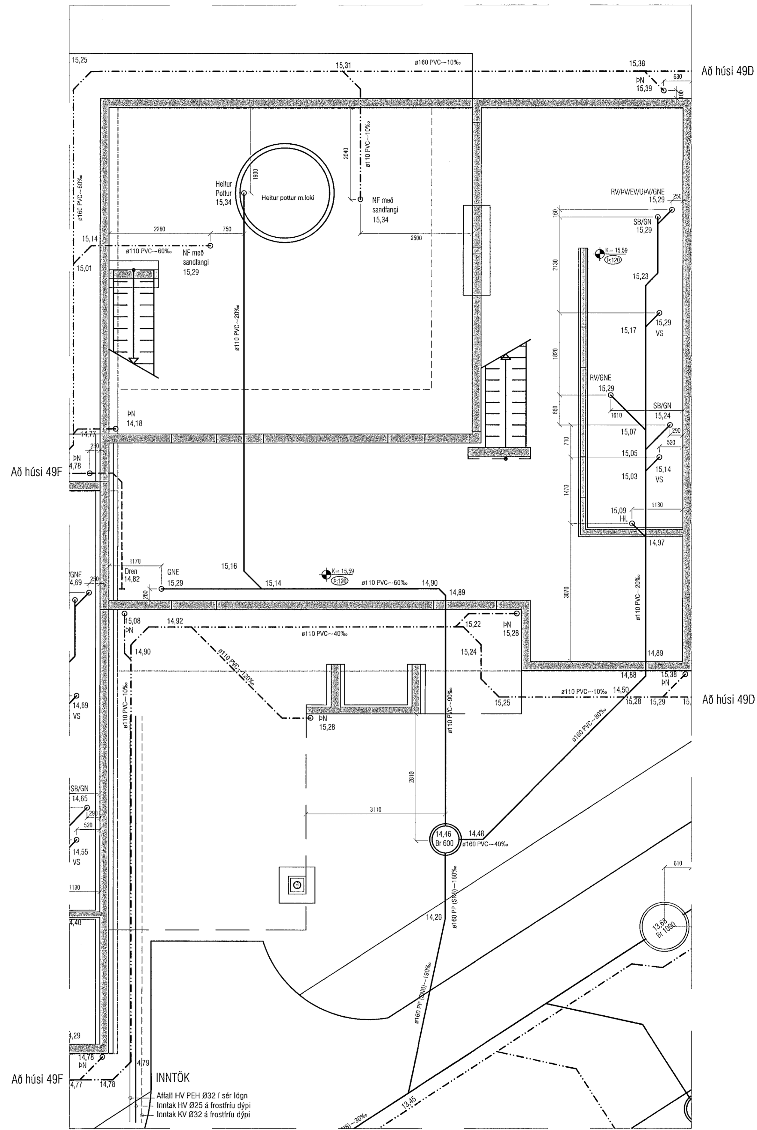
GRUNNMYND JARDLAGNA HÚS 49E
