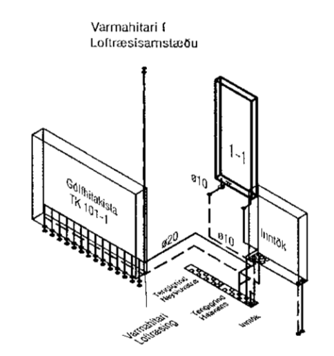
RÚMMYND HITLAGNA EINBÝLIHÚS LAGNIR ERU ÚR SVÖRTUM STÁLHRUM, SJÁ SKÝRINGABLAÐ LAGNA L-01
