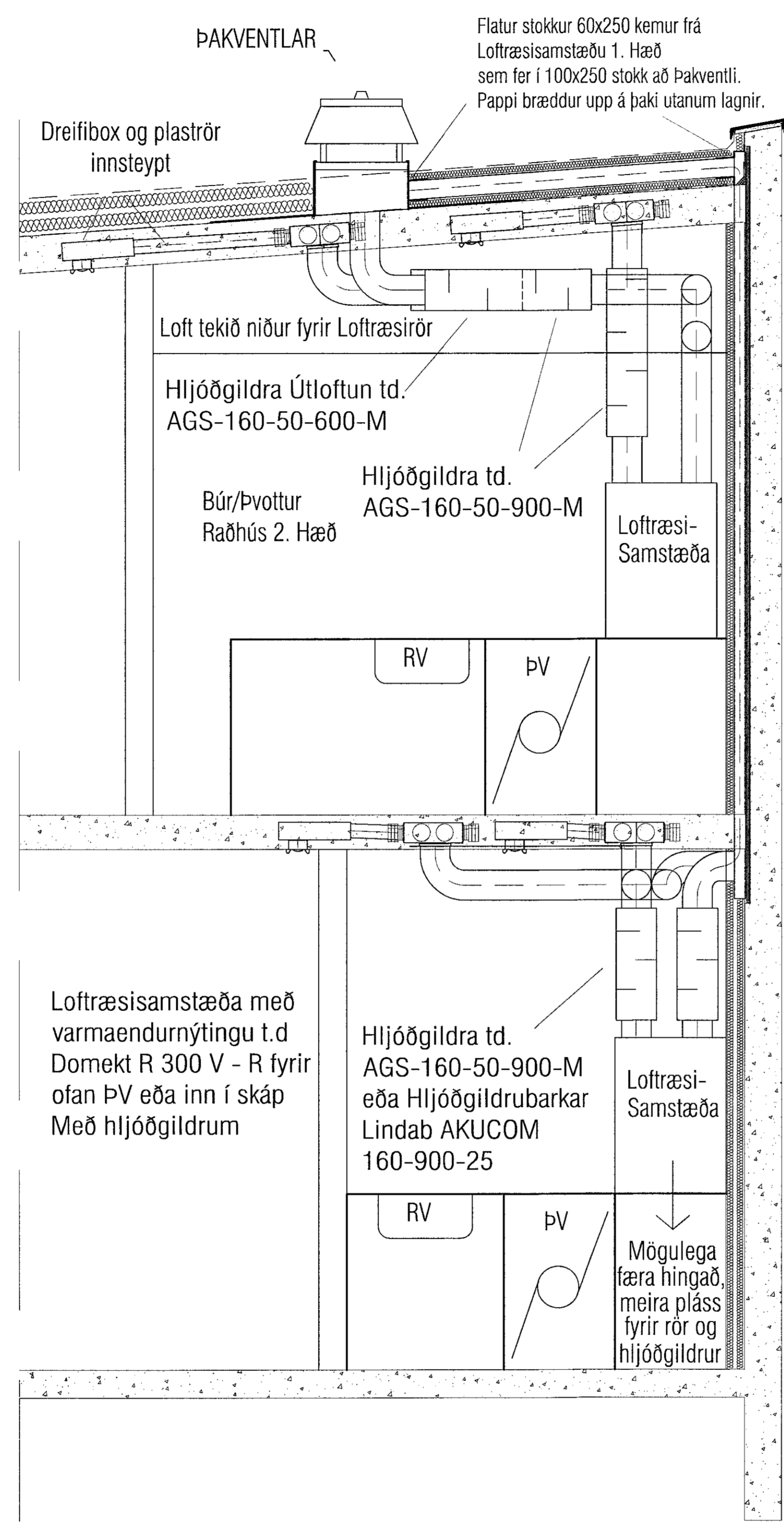
SNÍÐ LOFTRÆSING RADHÚS
