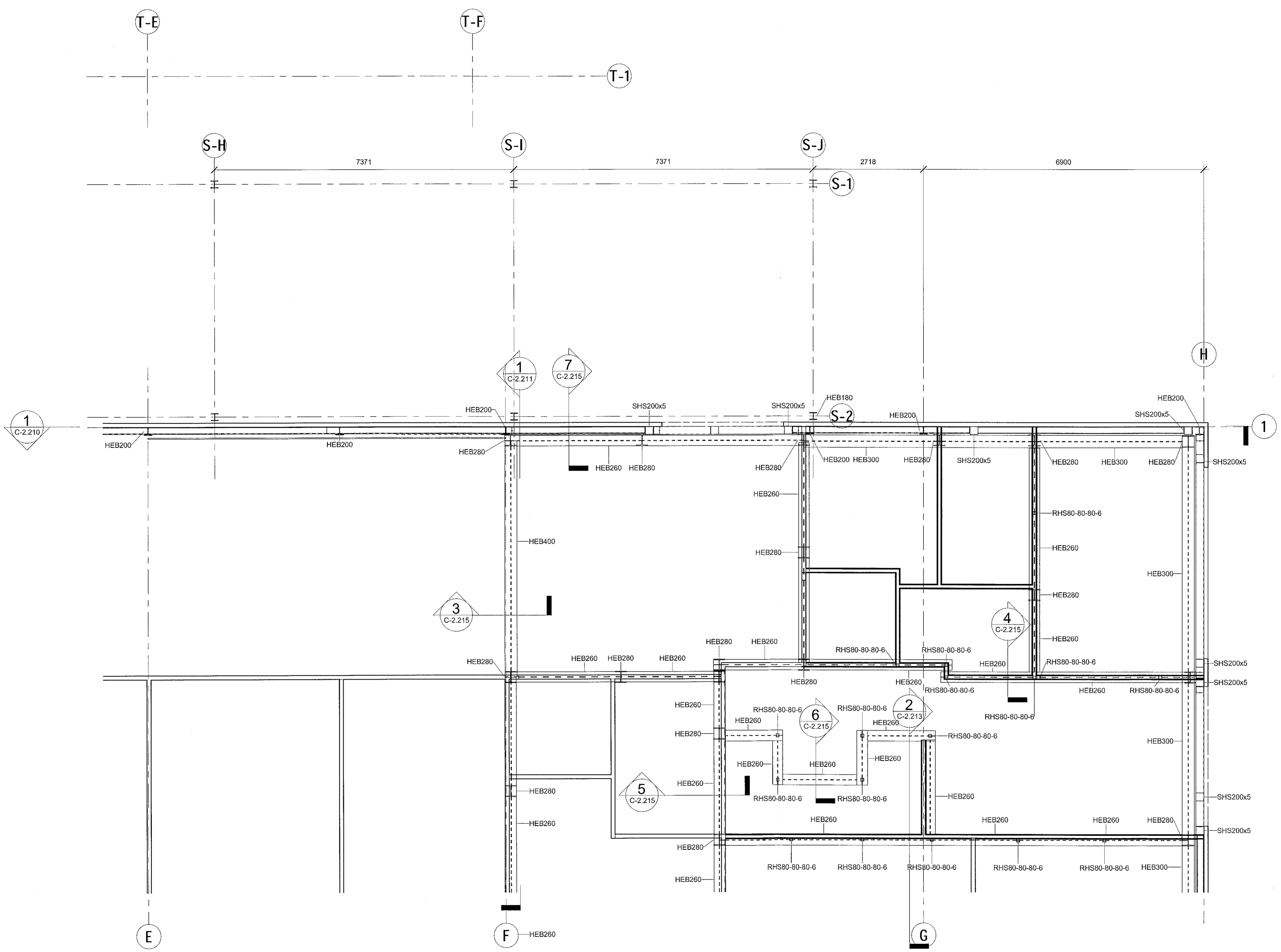
1.HÆÐ GRUNNMYND 5 AF 6 1 : 50
