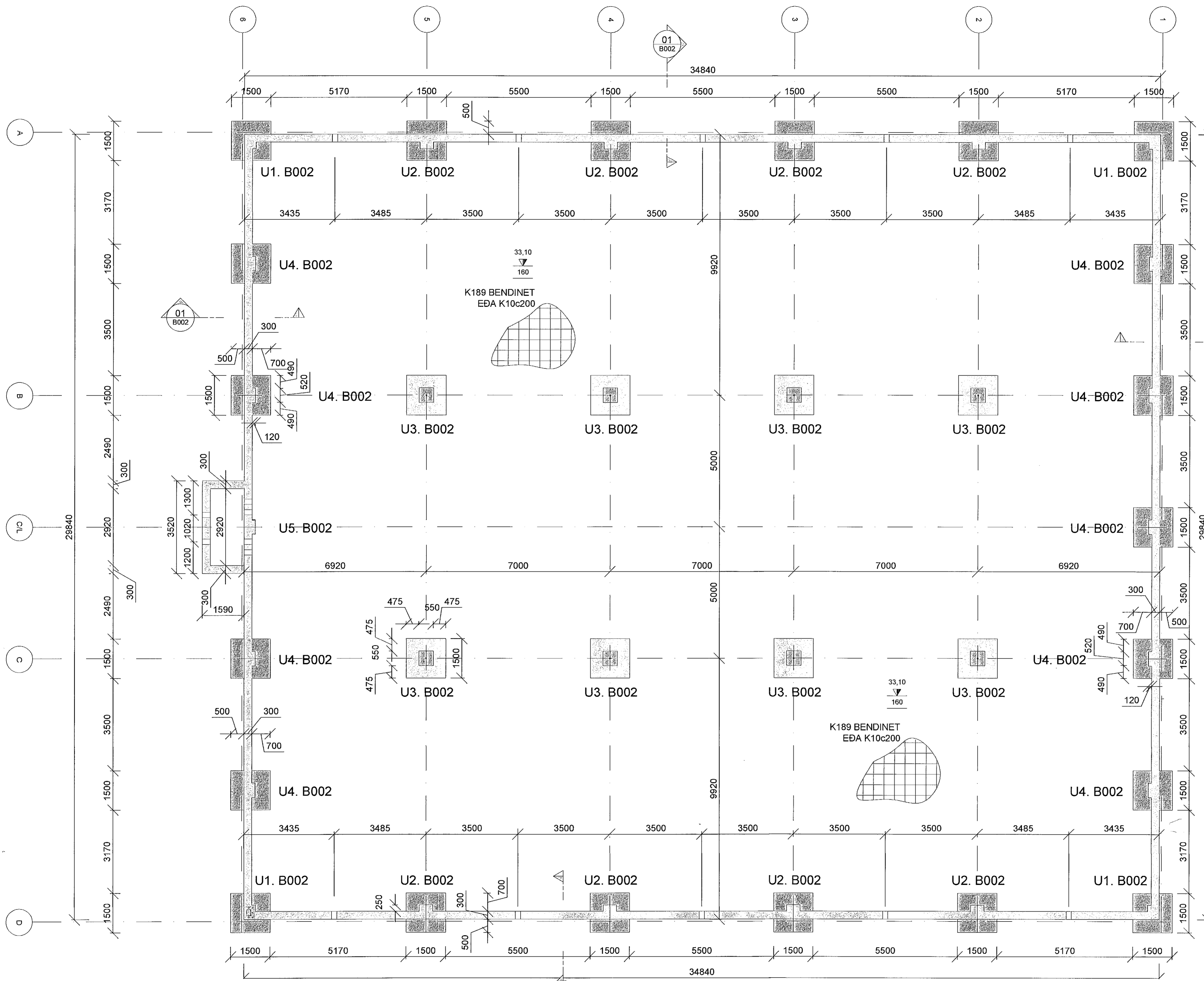
GRUNNMYND - UNDIRSTÖÐUR 1:75 (A1)
