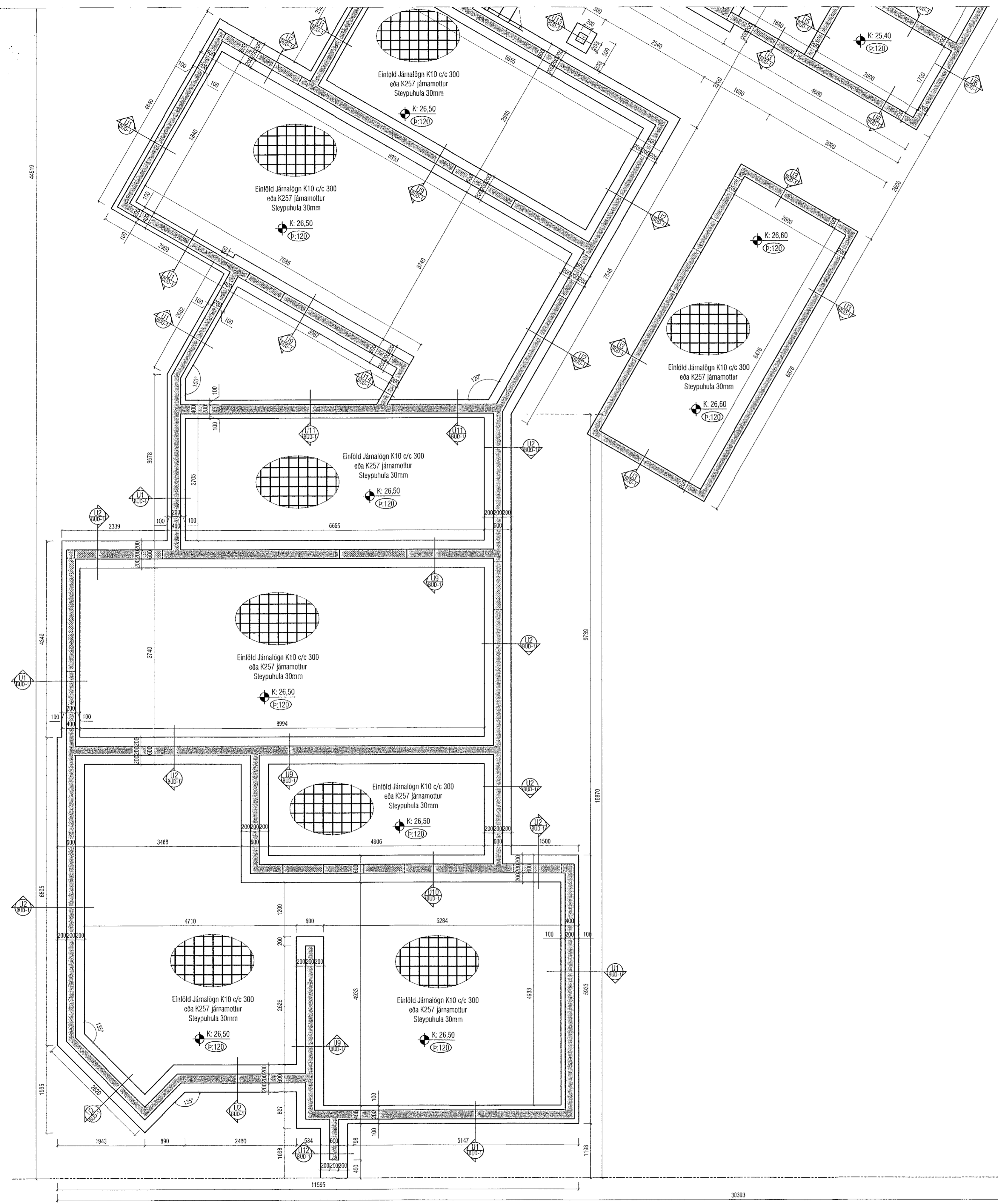
GRUNNMYND UNDIRSTADA MKV. 1:50
