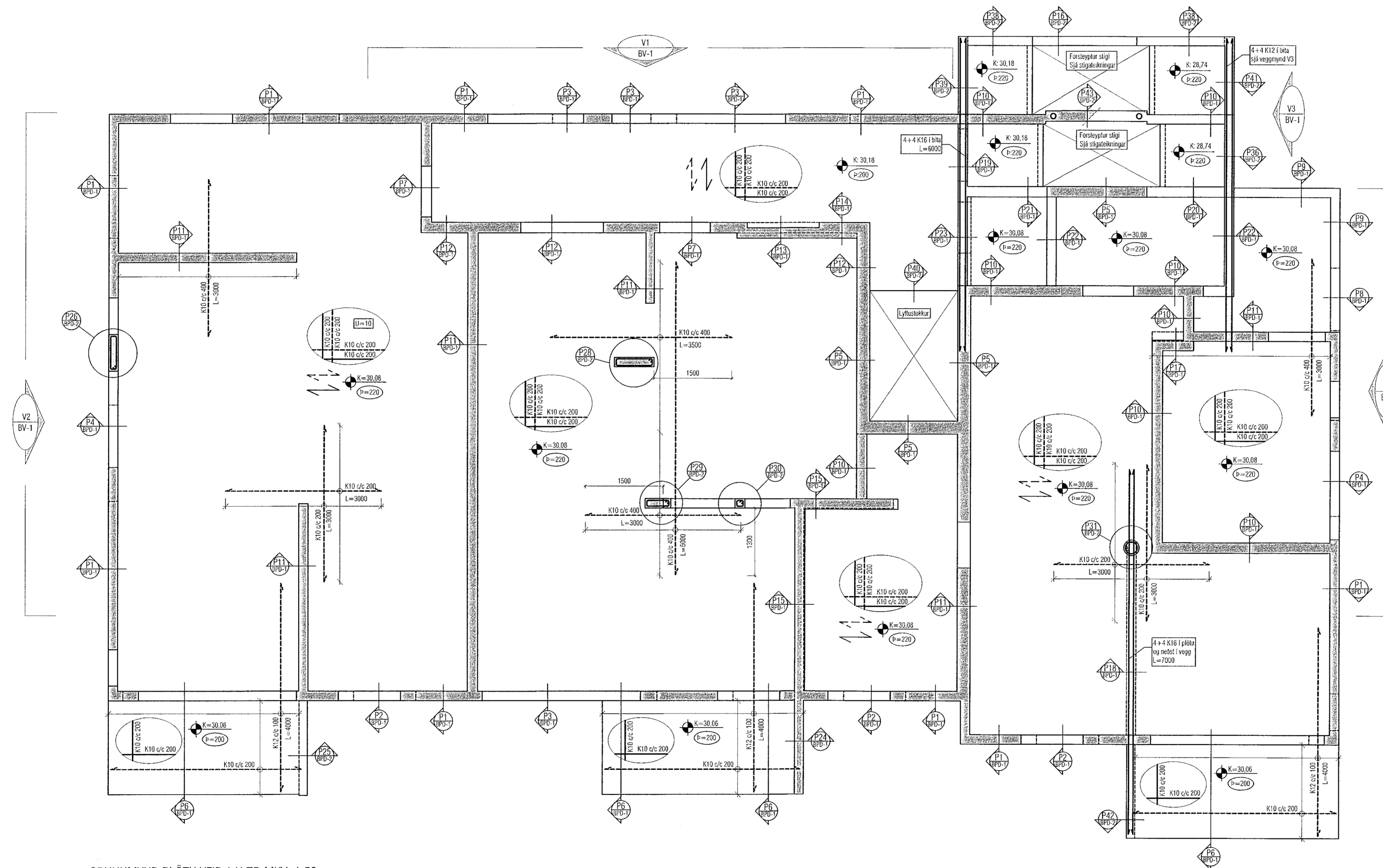
GRUNNMYND PLÖTU YFIR 1.HÆÐ MKV. 1:50
