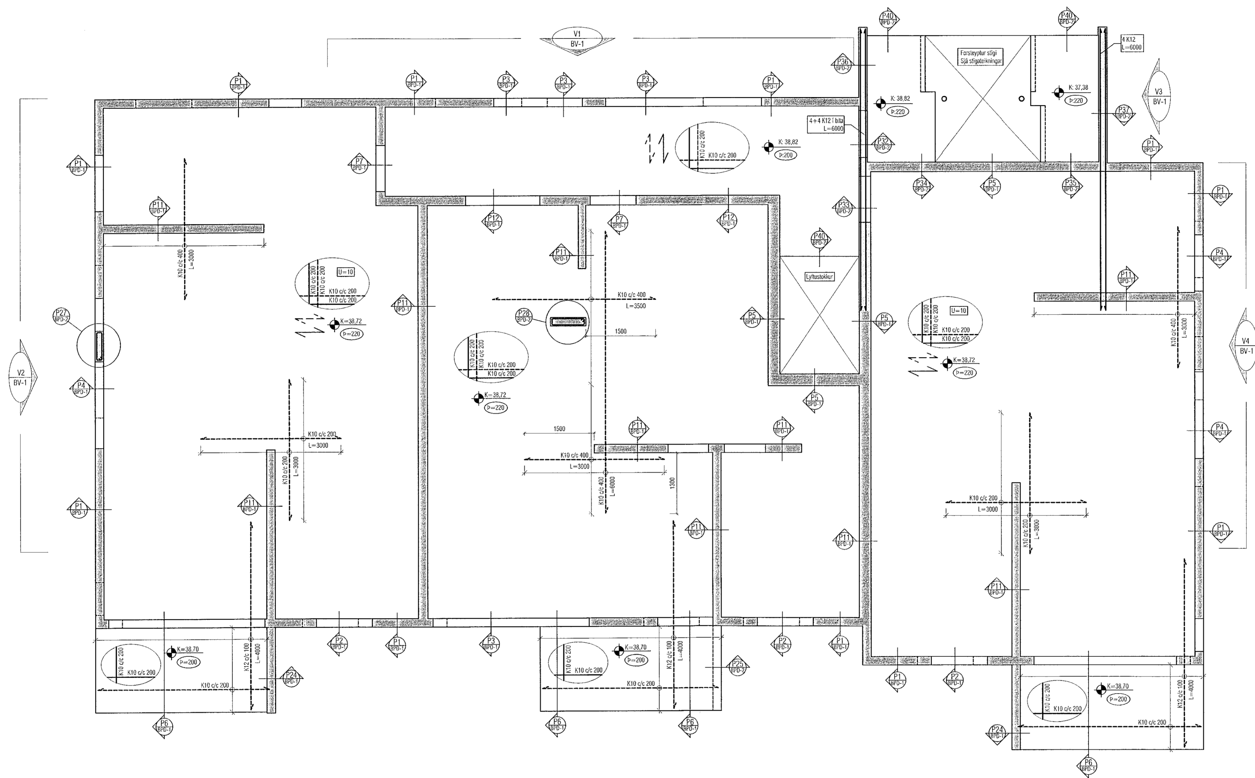
GRUNNMYND PLÖTU YFIR 4.HÆÐ MKV. 1:50
