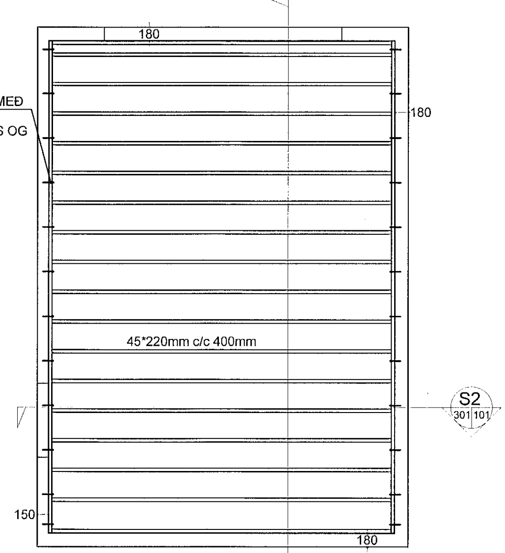
ÞAKVIRKI mkv. 1:50
