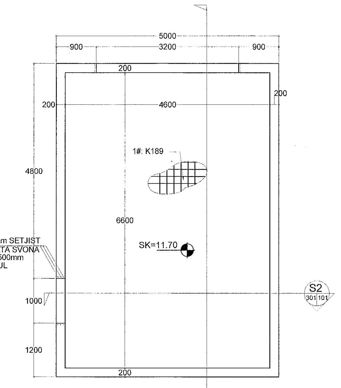
SÖKKULL mkv. 1:50
