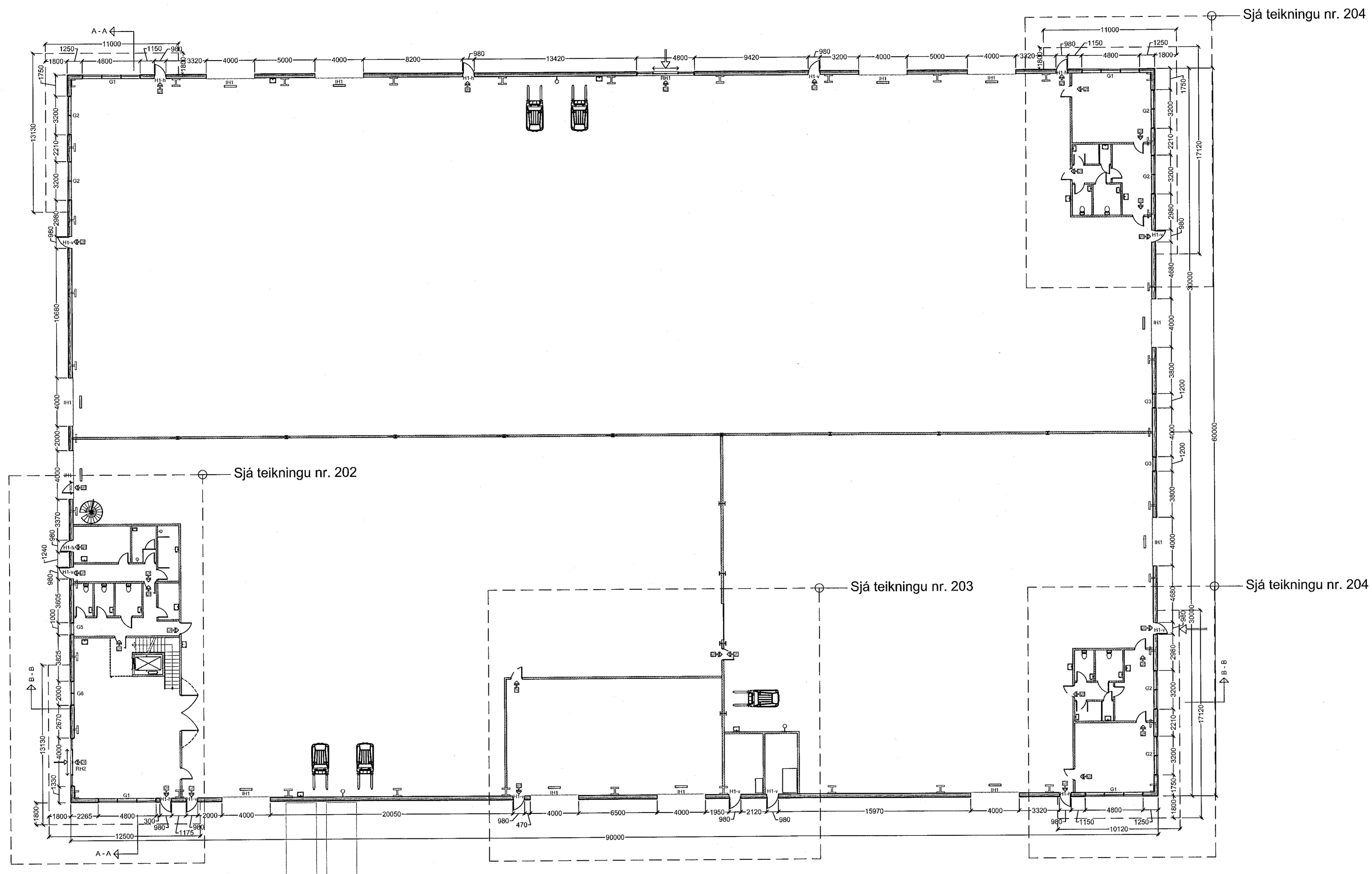
Grunnmynd 1 hæð mkv. 1:200 Yfirlitsmynd vinnuteikninga
