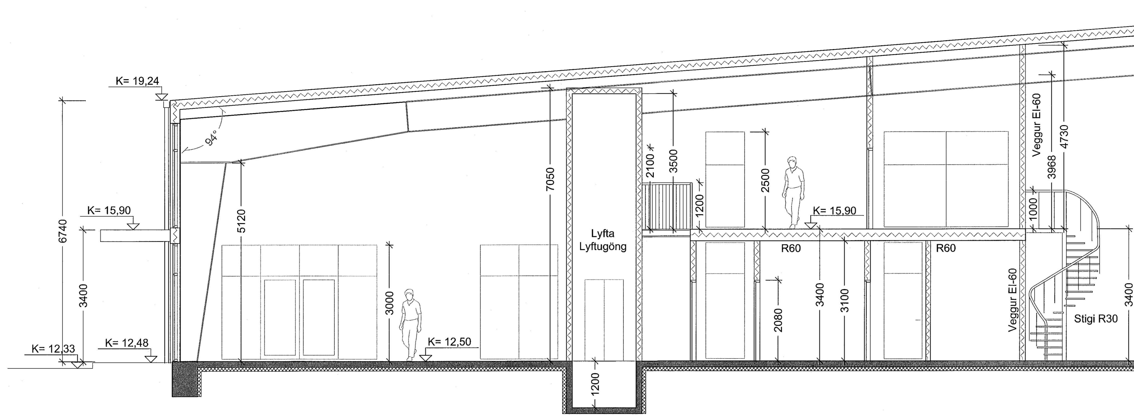
Sneiðing A - A mkv. 1:50
