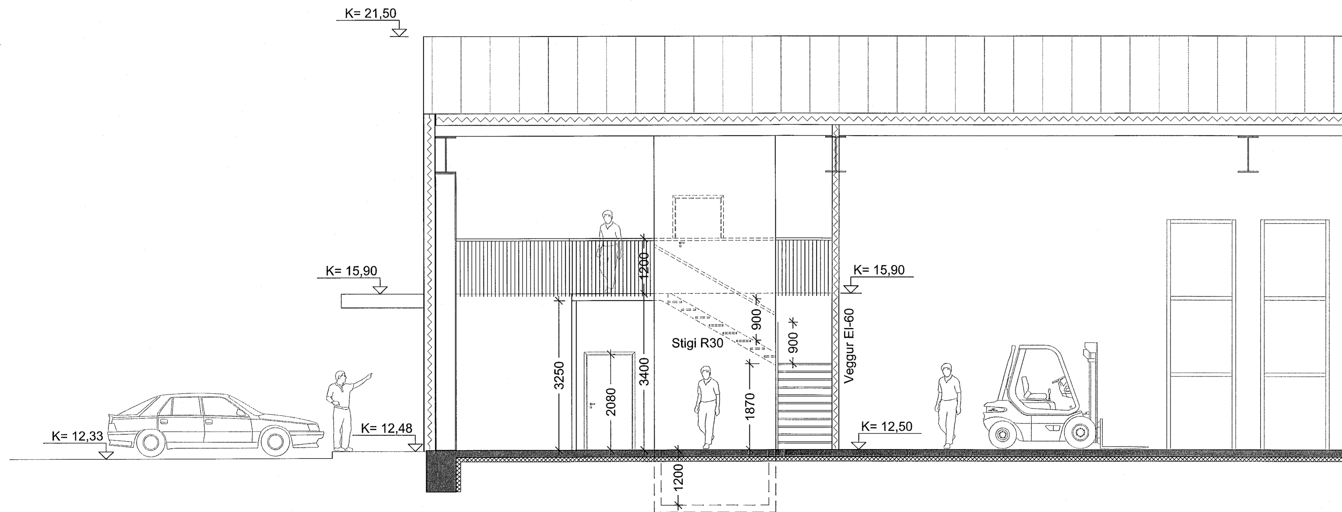
Sneiðing B - B mkv. 1:50
