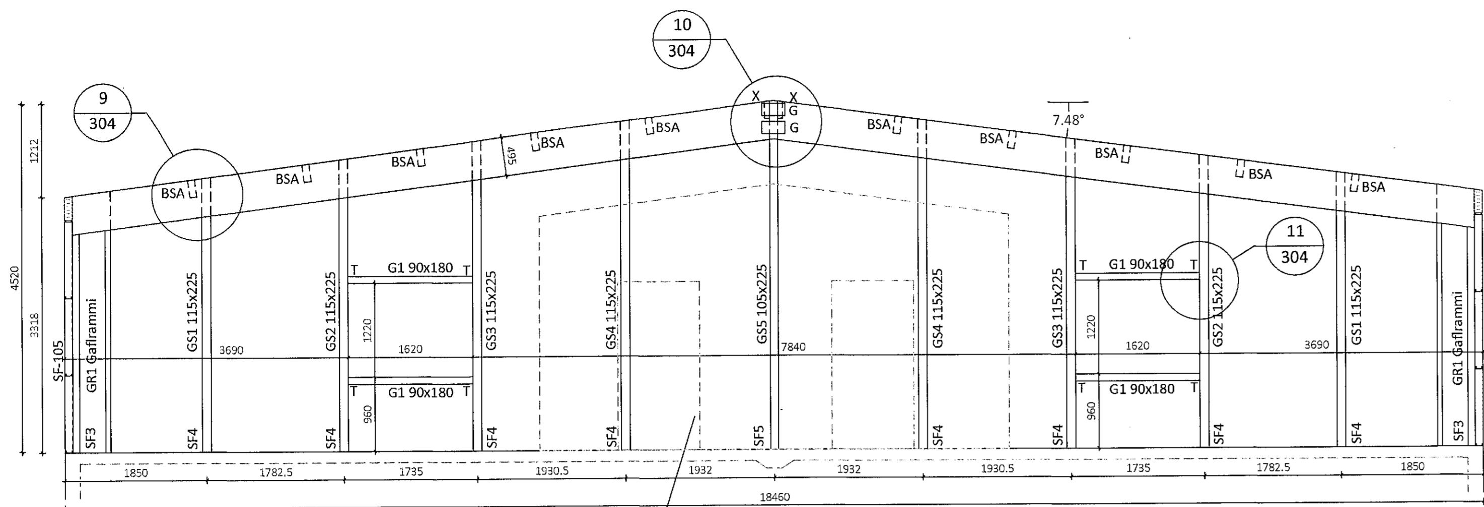
Ásýnd á suðaustur og norðvestur gaffl Mkv. 1:50 Límtré
