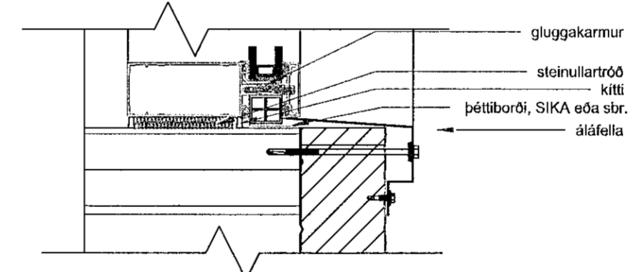
Frágangur ofan og neðan við glugga
