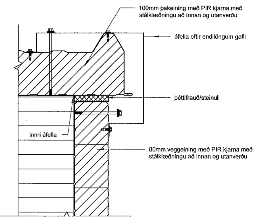
Frágangur við gafi
