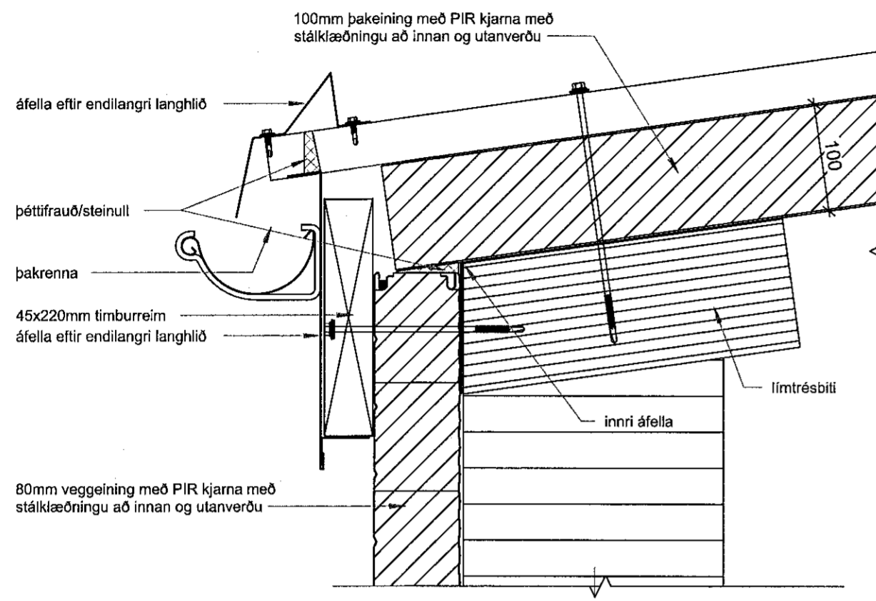
Frágangur við þakbrún
