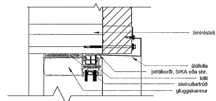
Frágangur við gafi
