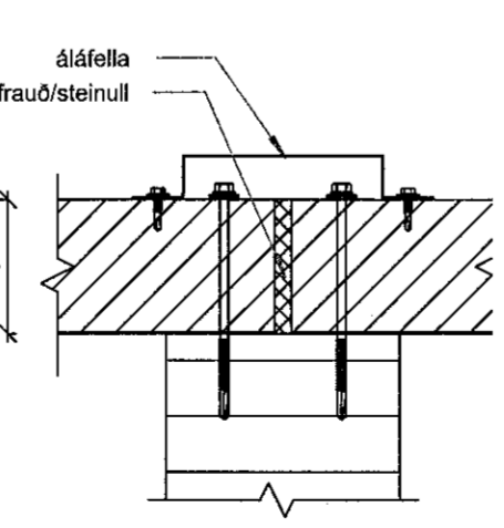
Frágangur við samskeyti veggjapanela
