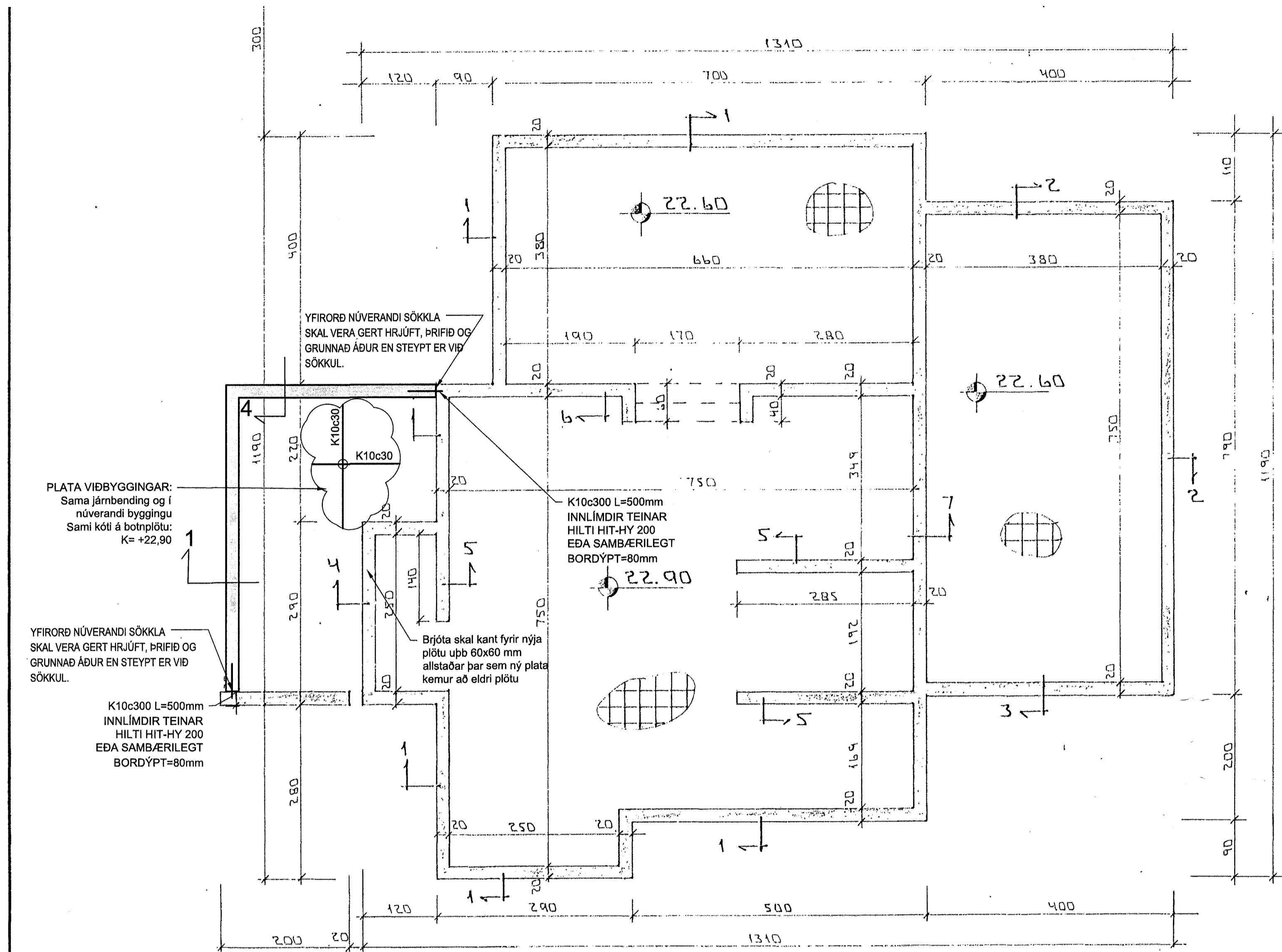
GRUNNMYND 1:50
