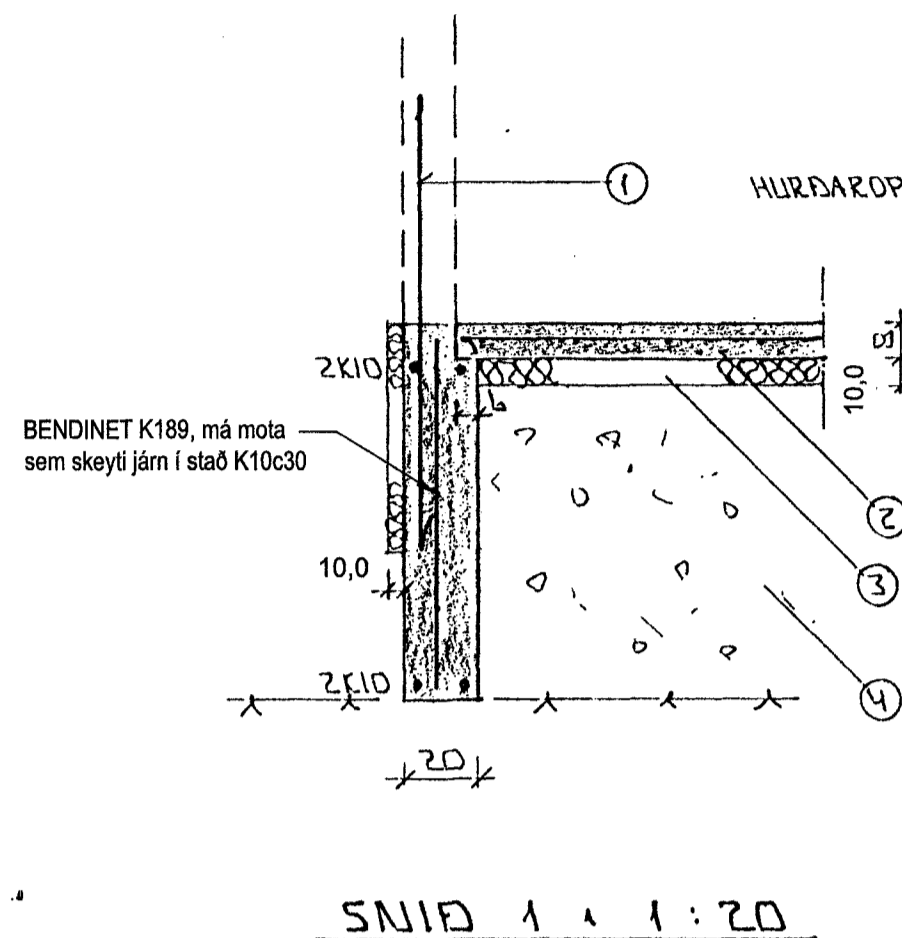
SNID 1:1:20
