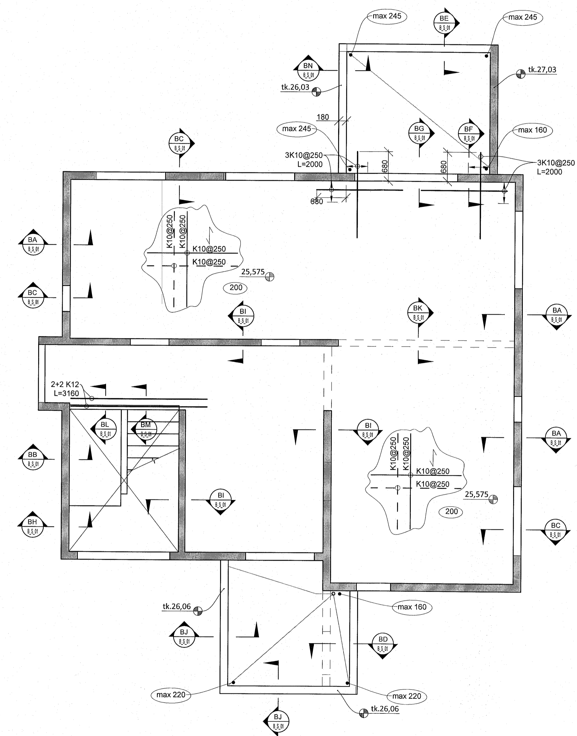
Grunnmynd - 2. hæð M 1:50
