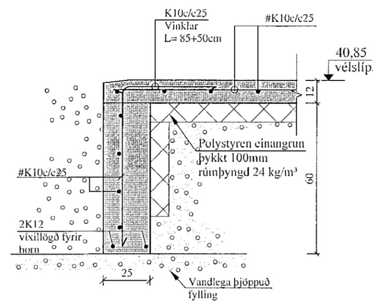
C3 SNID. 1:20 1-03 Útveggur
