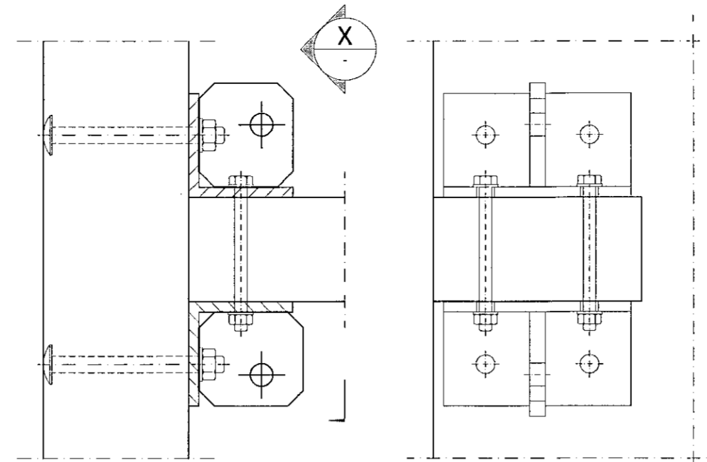
B1 Mkv. 1:5 Boltast saman með: 4 stk. borðboltum M16x180 2 stk. stálboltum M16x150
