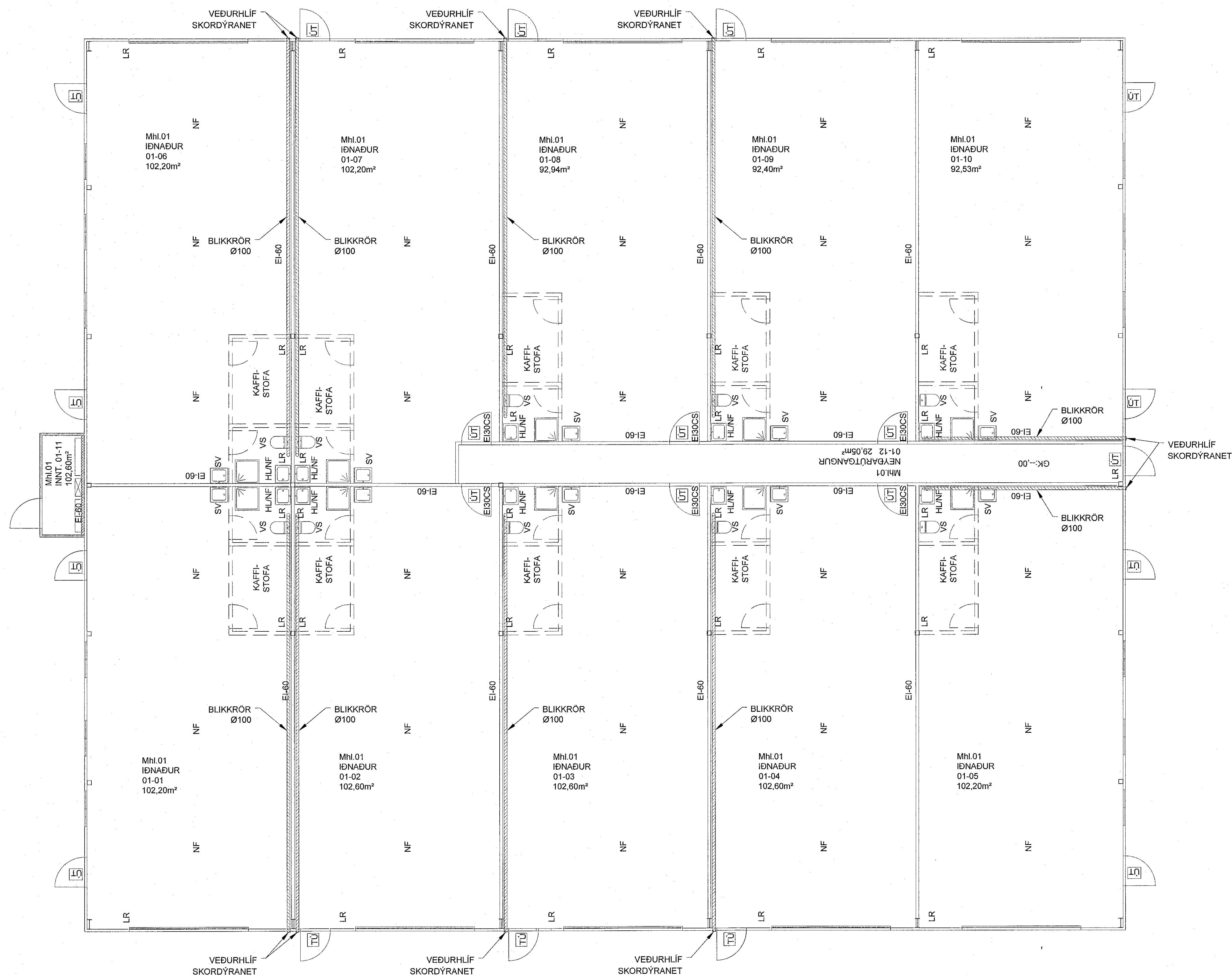
GRUNNMYND - LOFTRÆSTRILAGNIR 1:75 (A1)
