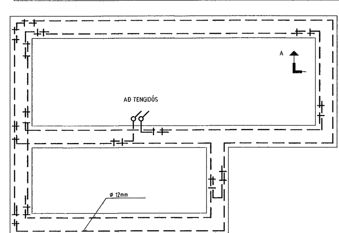
GRUNNMYND SÖKKULVEGGJA
