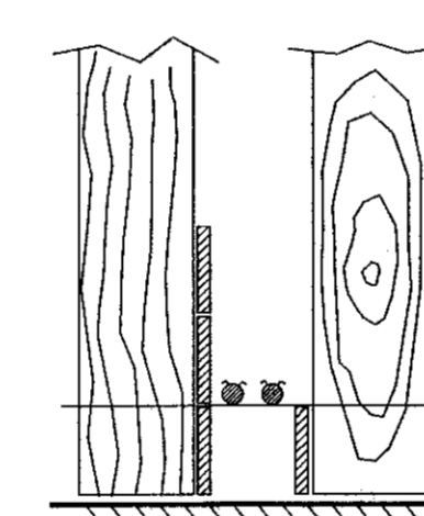
SNÍÐ A - A Í SÖKKULVEGG
