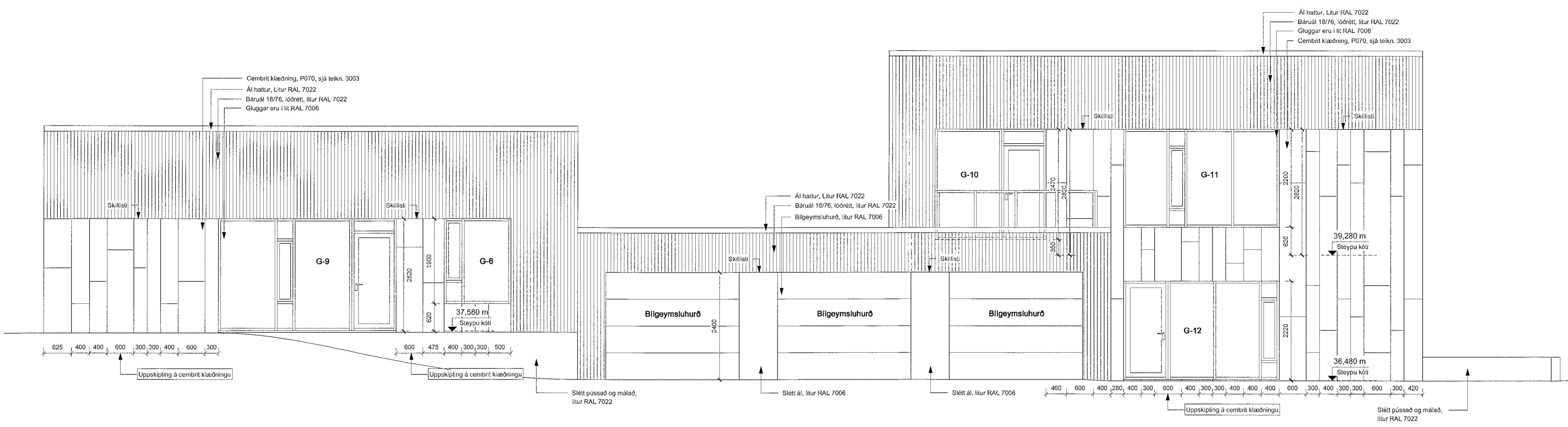
VERKT. - ÁSÝND SUÐUR mkv: 1 : 50
