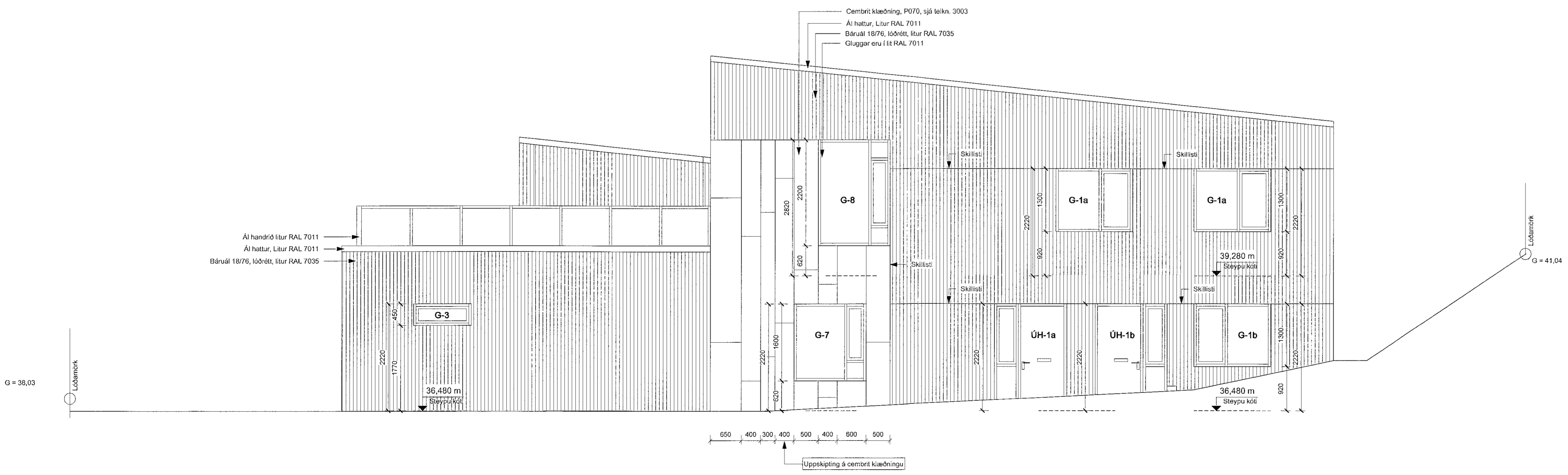
VERKT. - ÁSÝND AUSTUR mkv: 1 : 50
