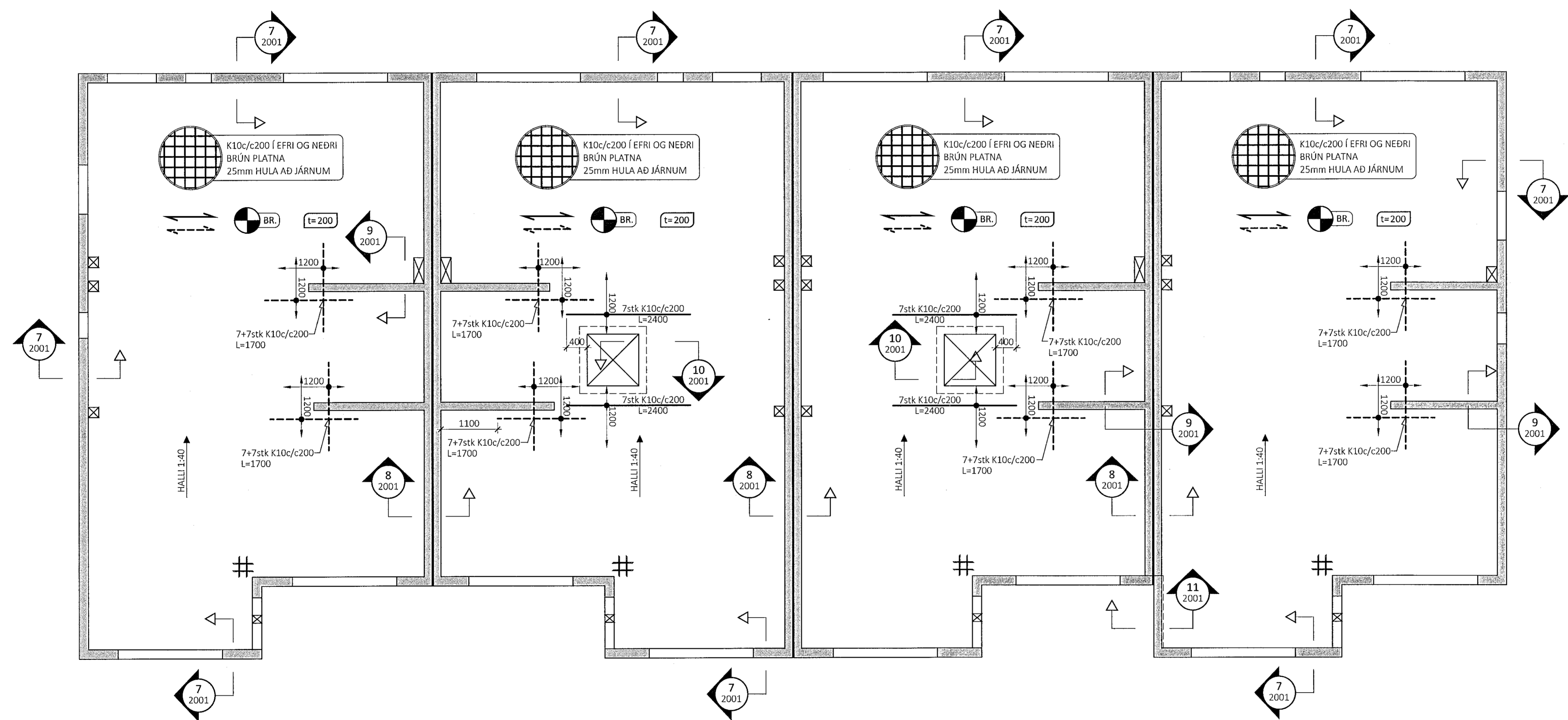
GRUNNMÝND PLÖTU YFIR 2. HÆÐ (ÞAKPLATA) - HÚS D TIL G - M1:50
