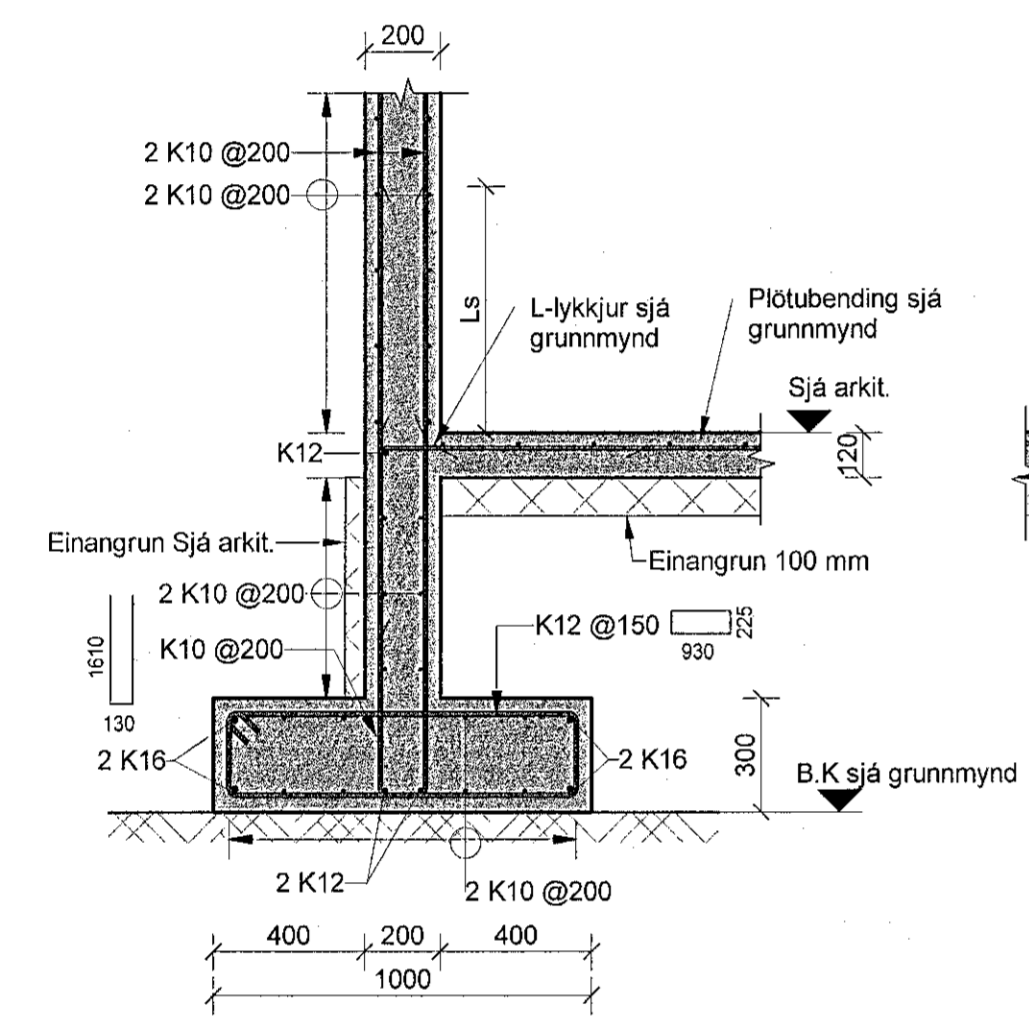
BF Snið BF -1,1,21,01 1 : 20
