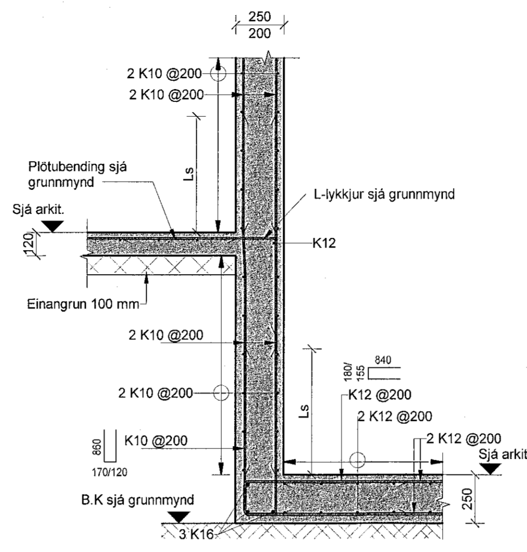
BC Snið BC -1,1,21,01 1 : 20
