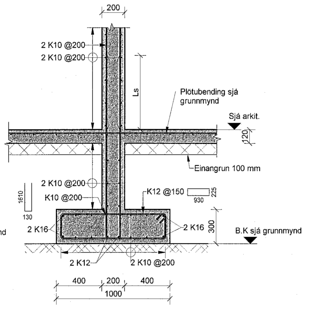
BG Snið BG -1,1,21,01 1 : 20
