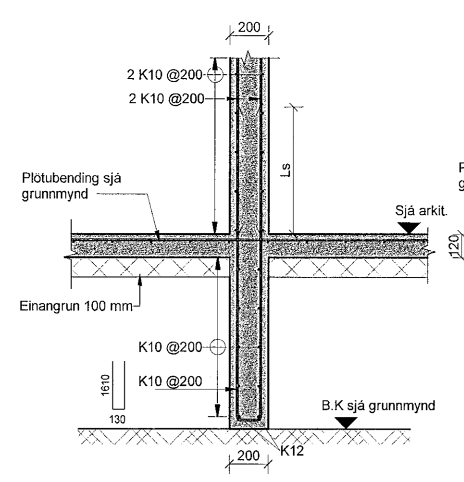
BD Snið BD -1,1,21,01 1 : 20
