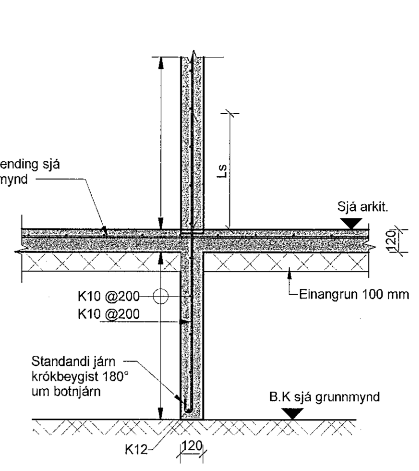
BE Snið BE -1,1,21,01 1 : 20
