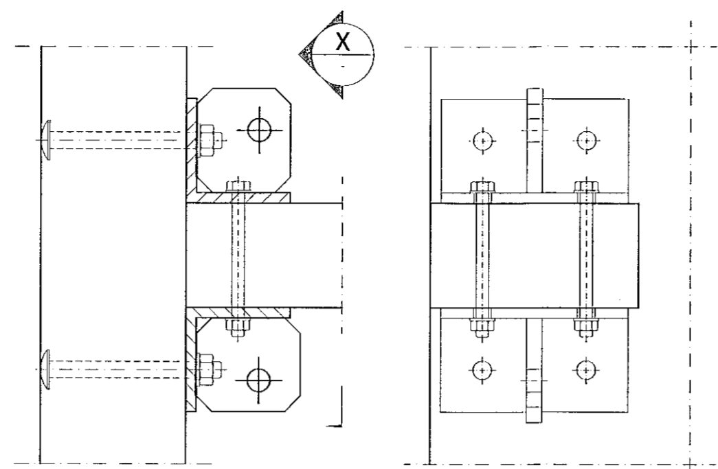
Boltast saman með: 4 stk. borðboltum M16x180 2 stk. stálboltum M16x150
