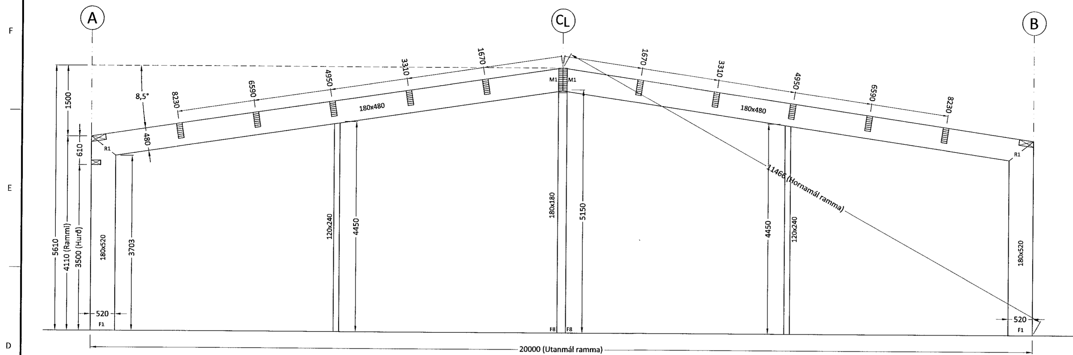
MODULE - 2-5 Mkv. 1:50
