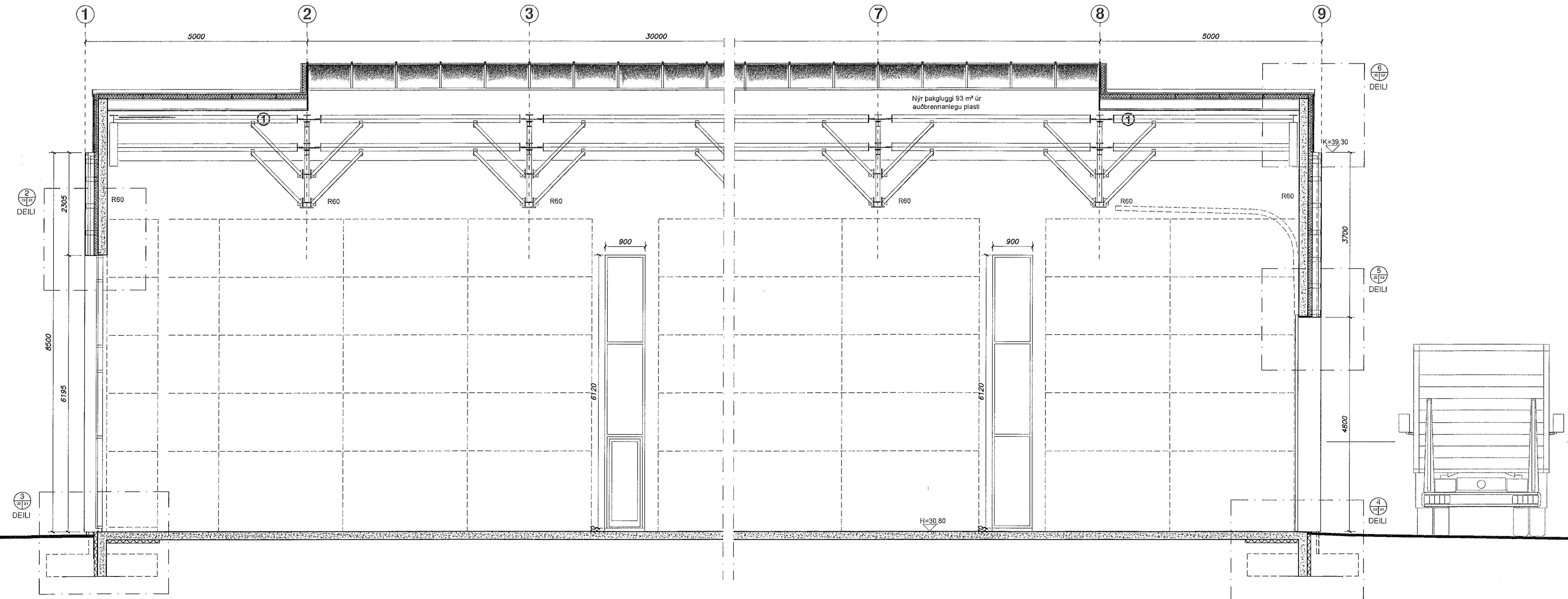
SNID C-C (hlutasnið) mkv. 1:50
