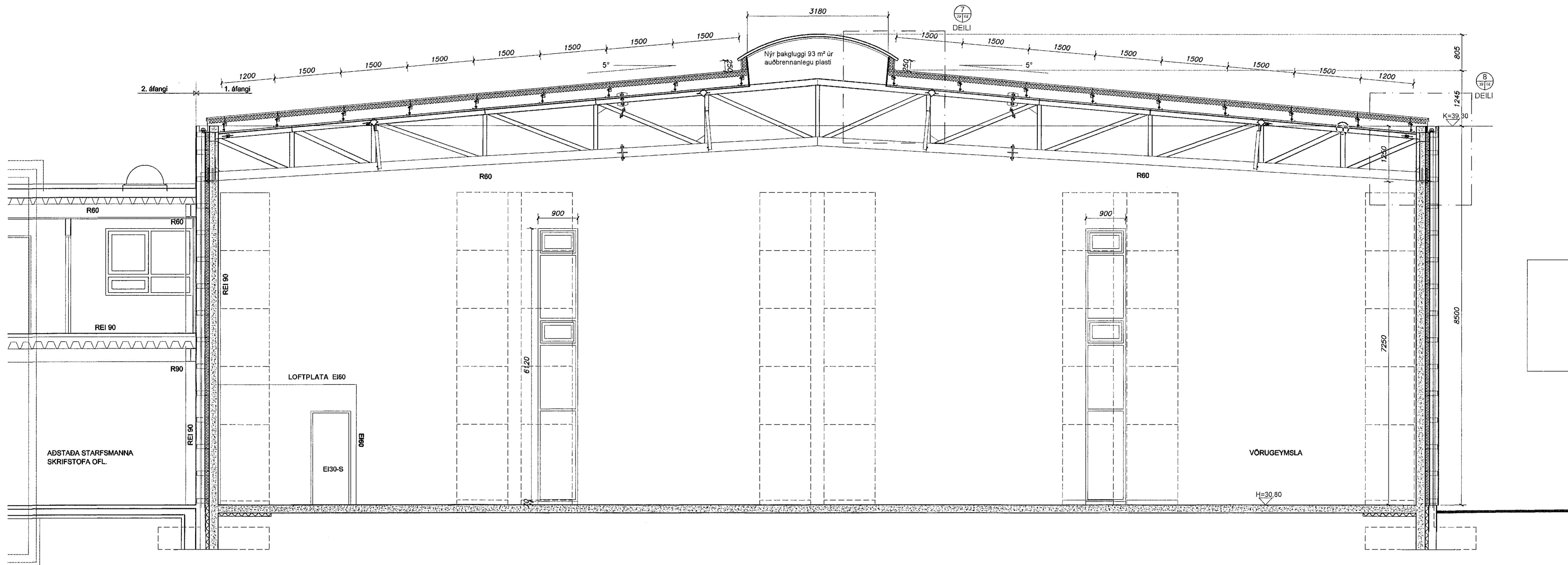
SNID A-A mkv. 1:50
