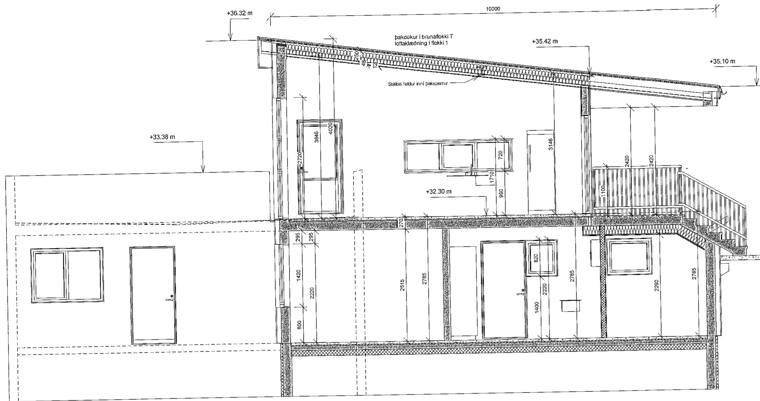
Sneiðing A Vinnut. 1 : 50
