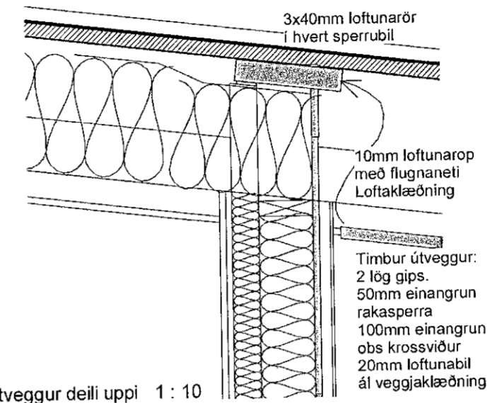
Léttur útveggur deili uppi 1 : 10
