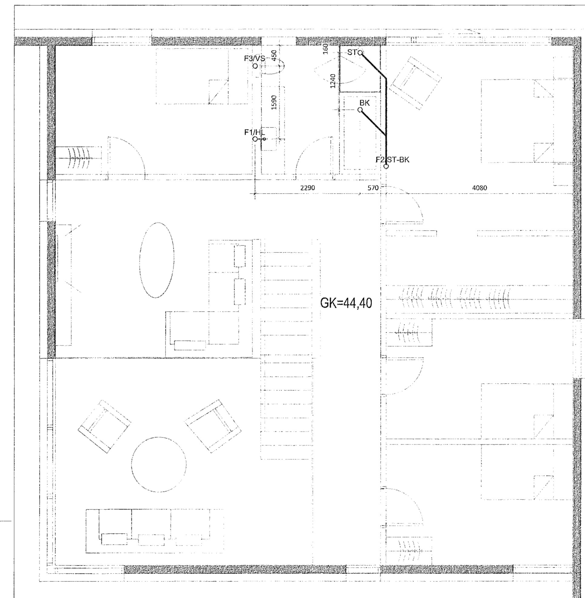
Grunnmynd frárennslis - 2.hæð MKV. 1:50
