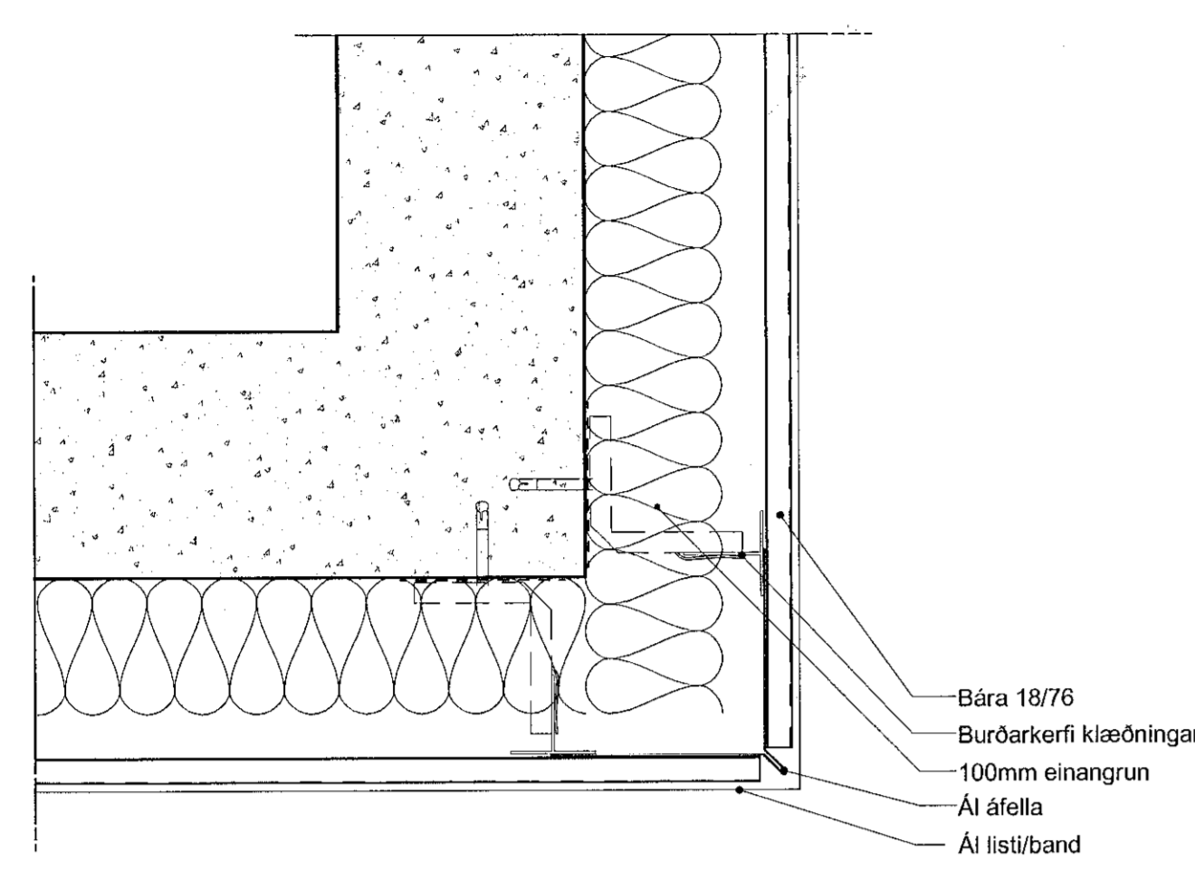
D-13- Lárétt 2.01-12
