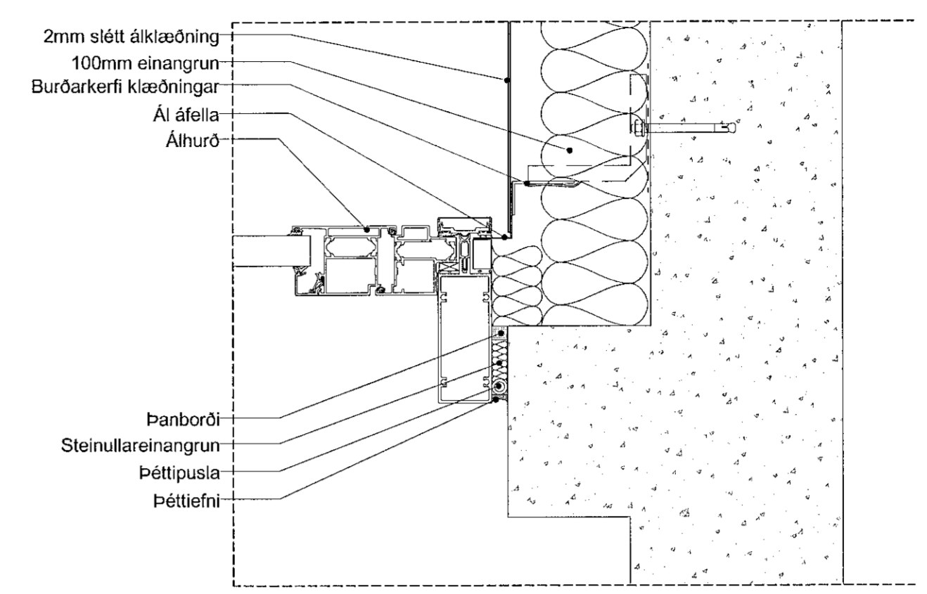
D-15- Lárétt 2.01-11
