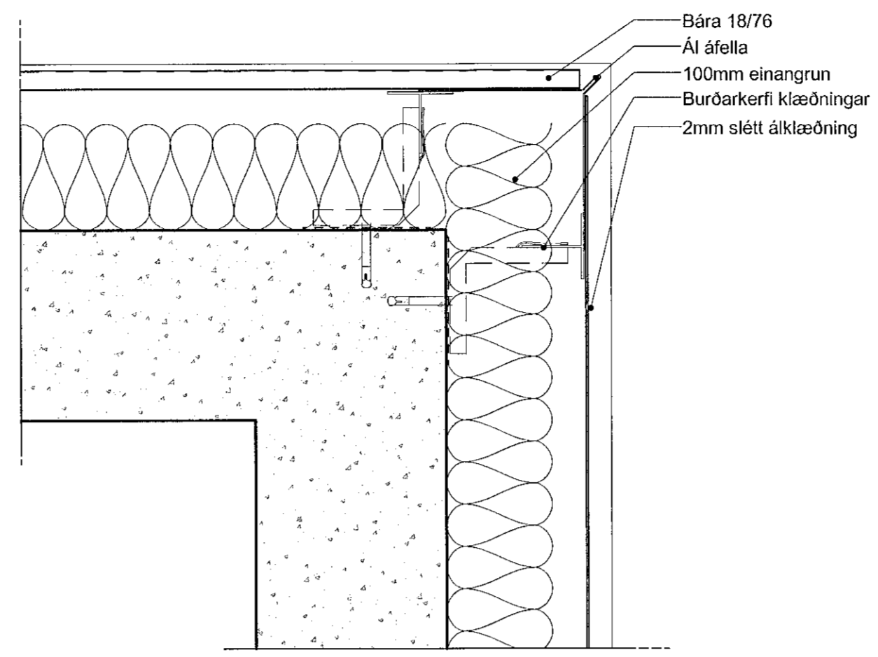
D-14- Lárétt 2.01-12
