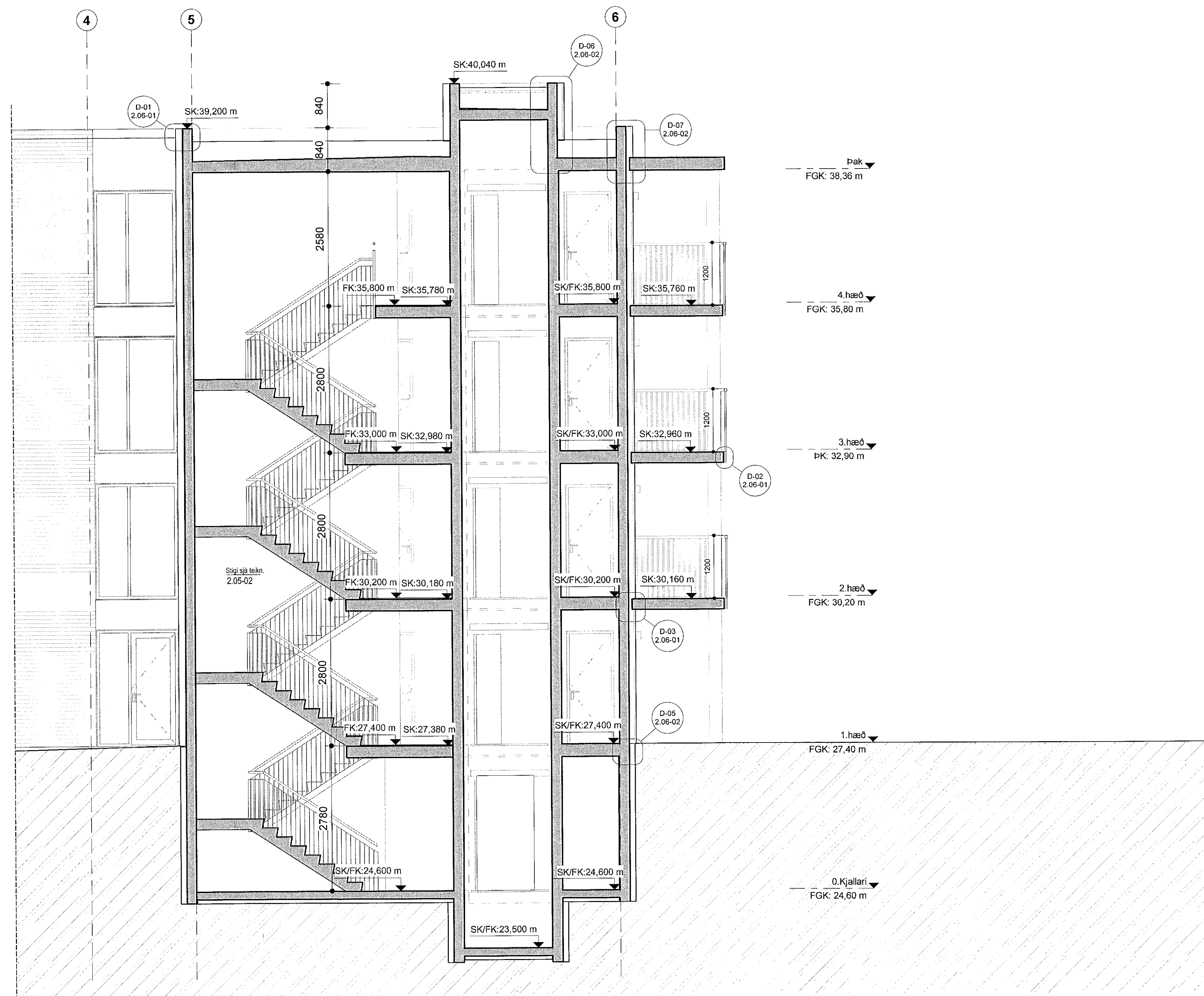
Snið B-B
