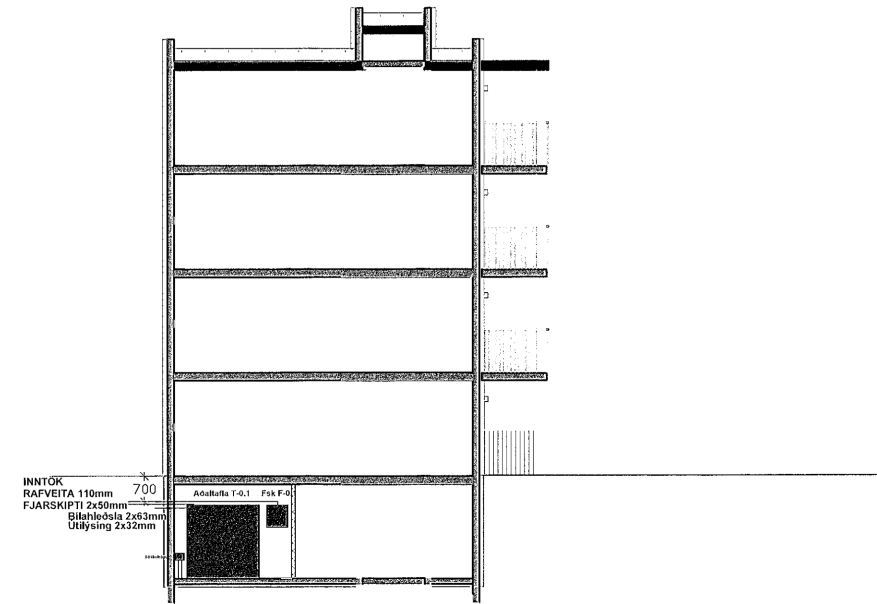
Sniðmynd 1:100
