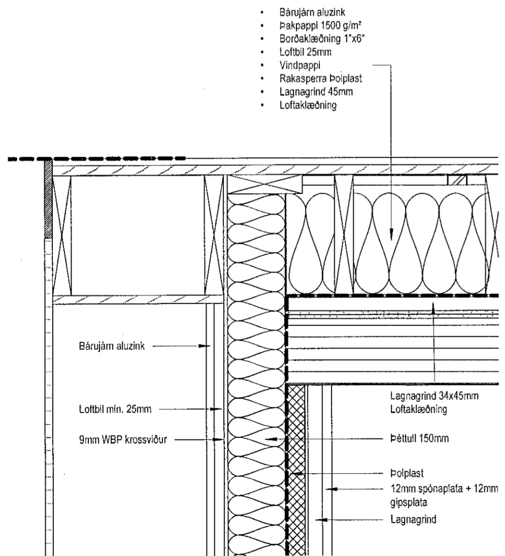
Deili 4 - A404 1 : 10
