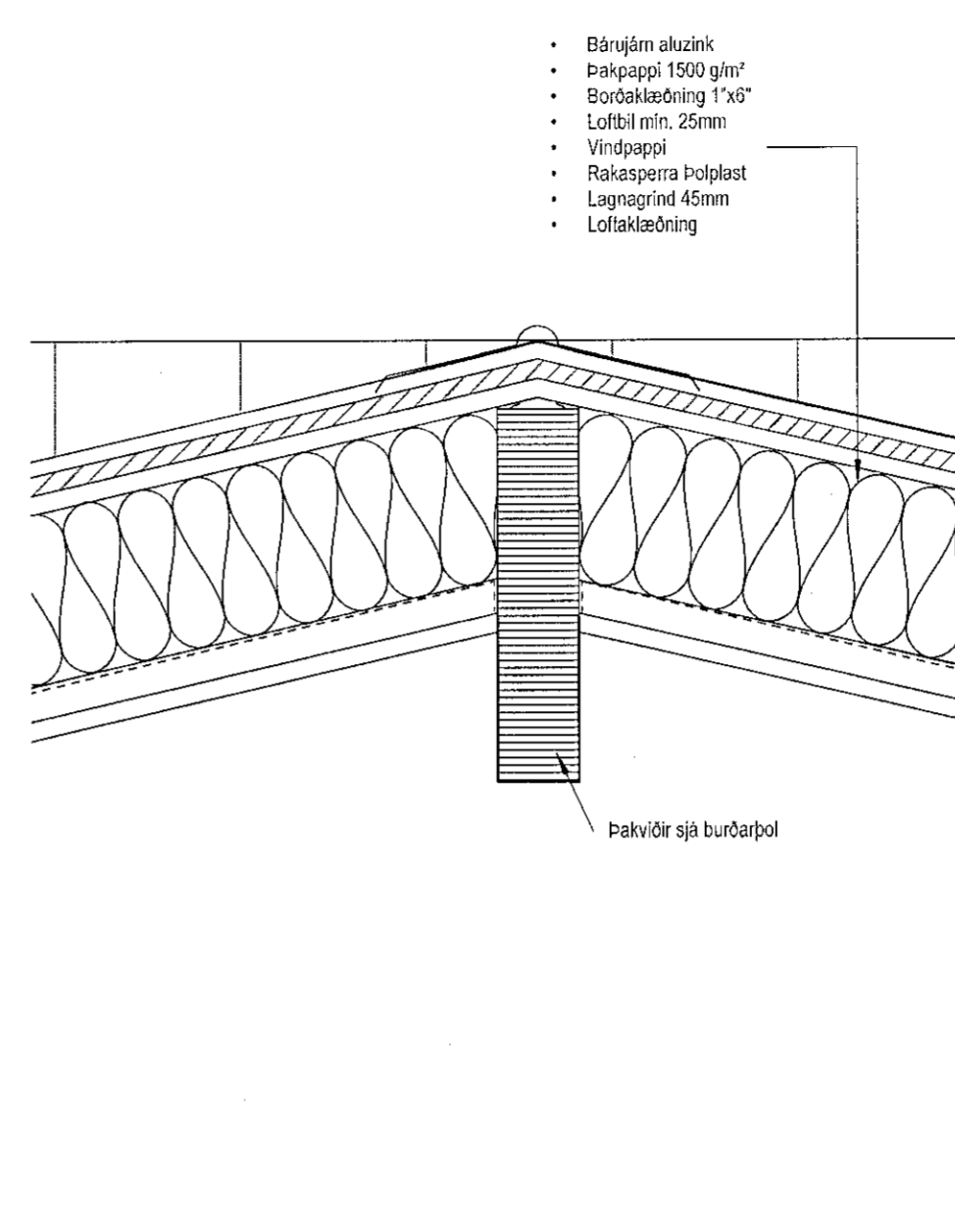
Deili 3 - A404 1 : 10
