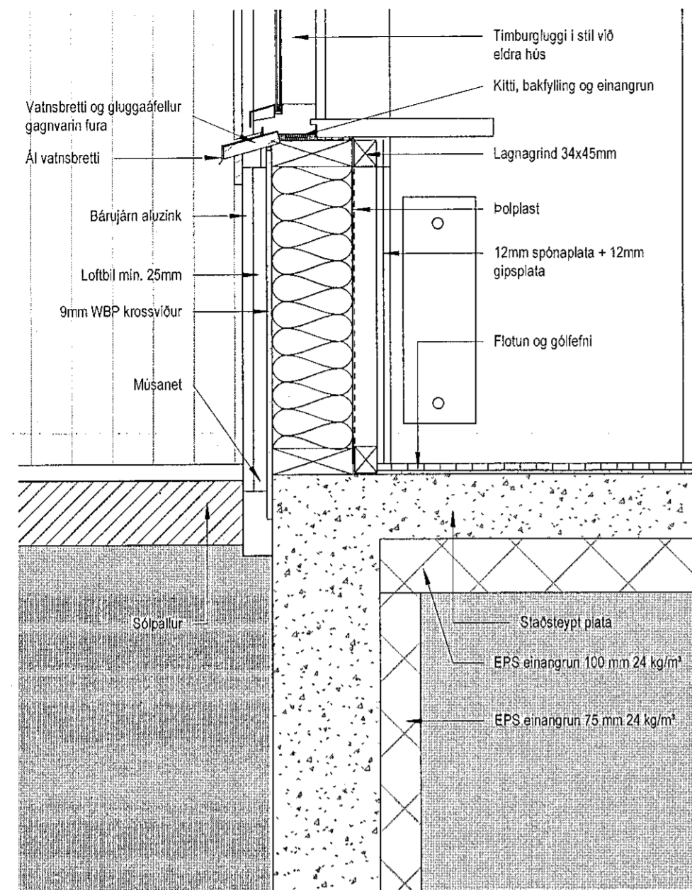
Deili 1 - A404 1 : 10
