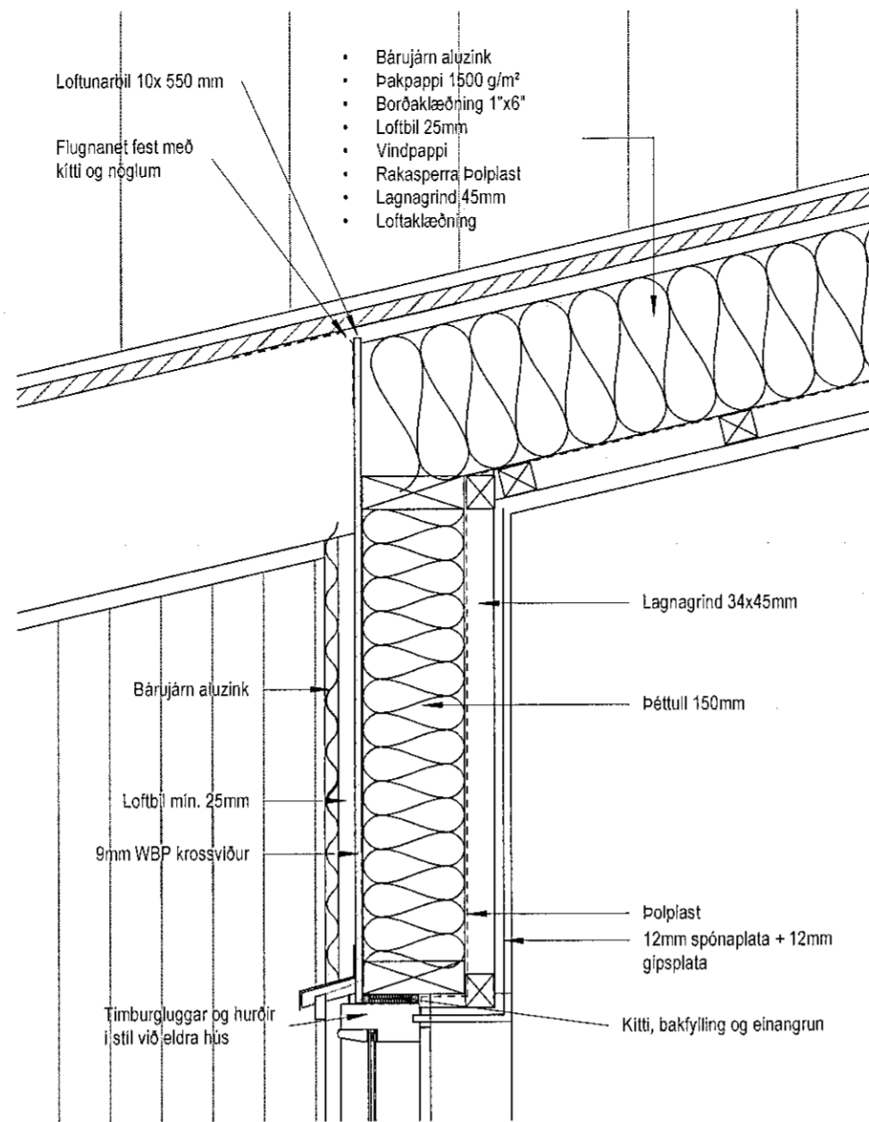
Deili 2 - A404 1 : 10
