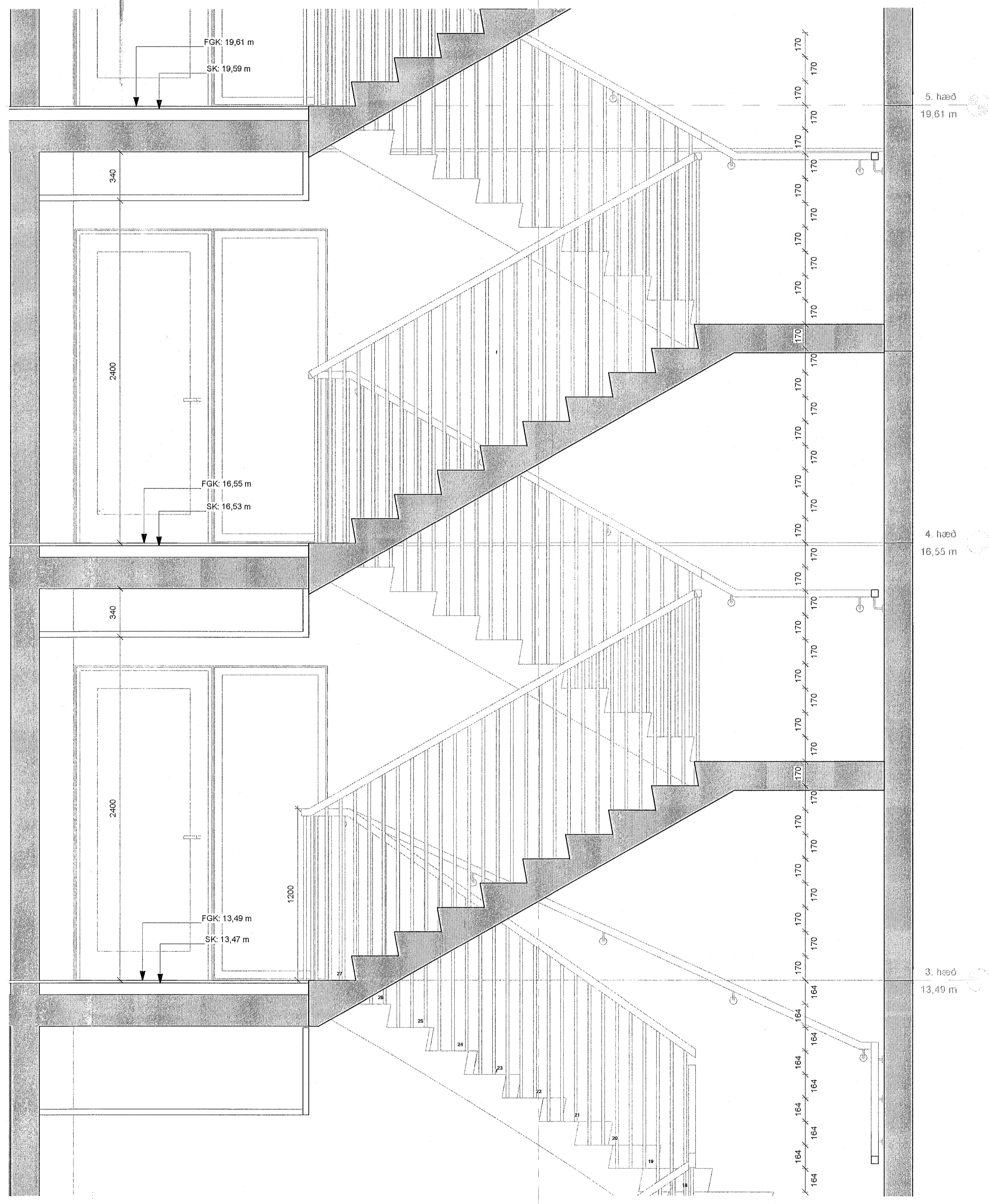
B2 Snið B-B - Stigahús nr.2 - 3-5 hæð 1 : 20
