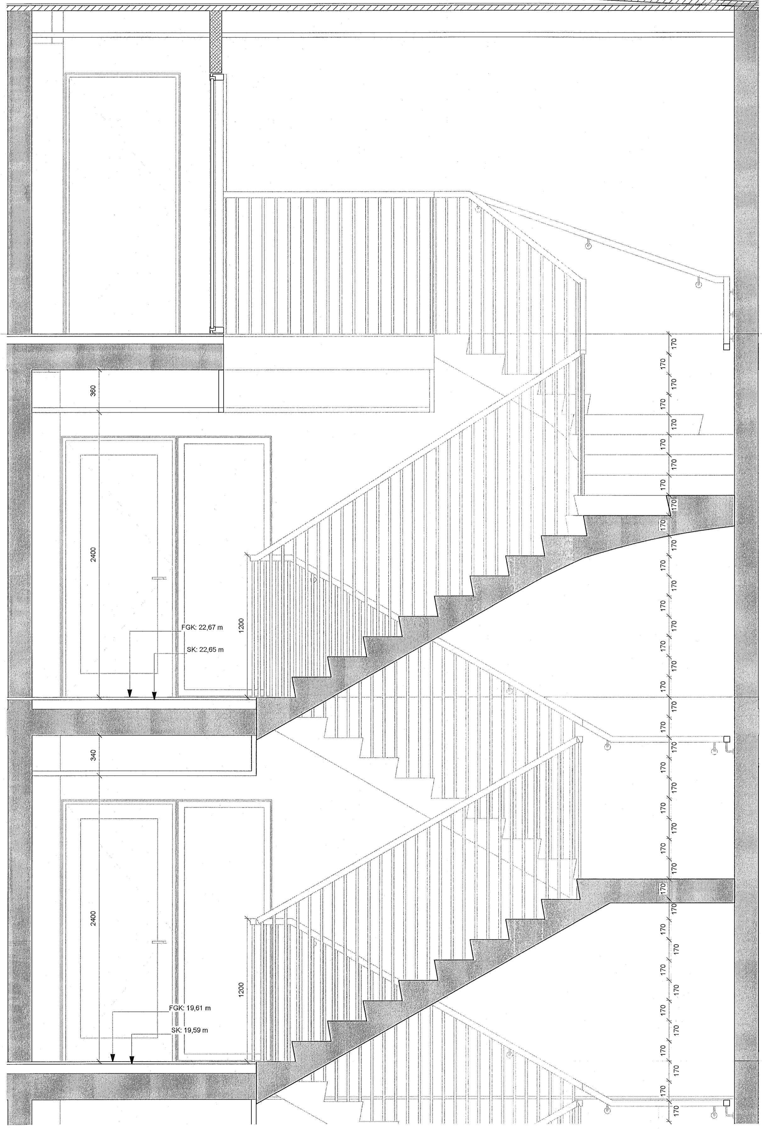
B1 Snið B-B - Stigahús nr.2 - 5-7 hæð 1 : 20
