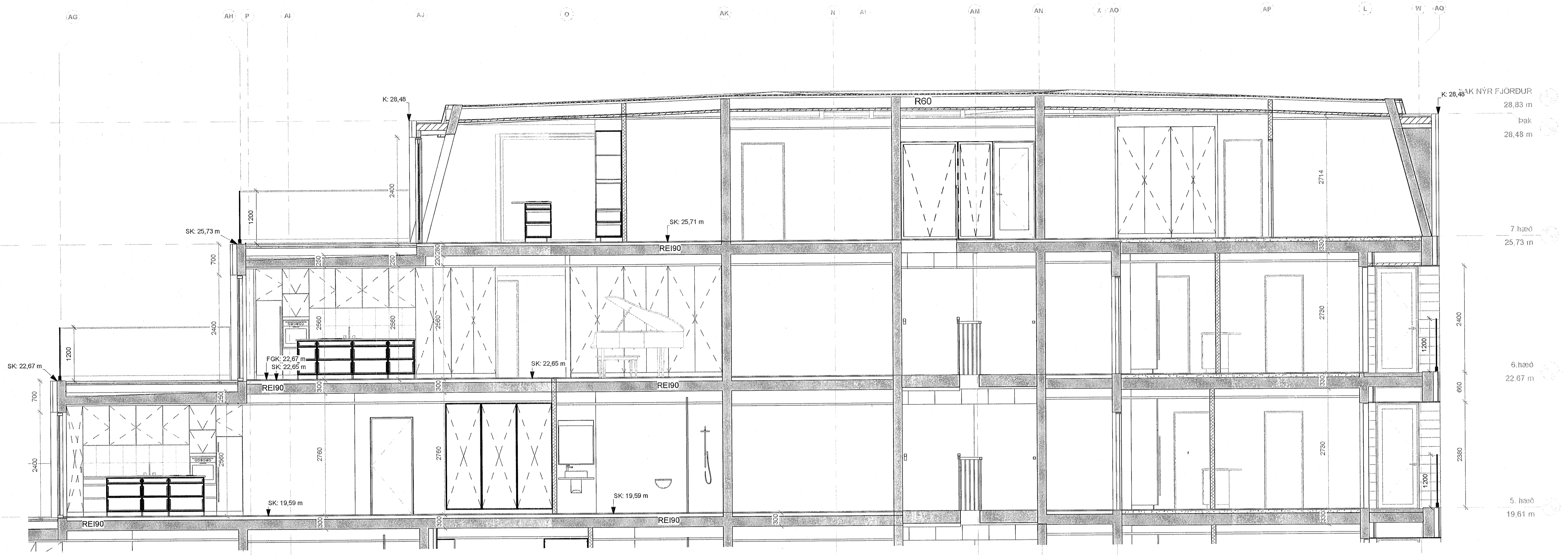
I-I 03 Sneiðing - Verk. I-I - 03 1 : 50
