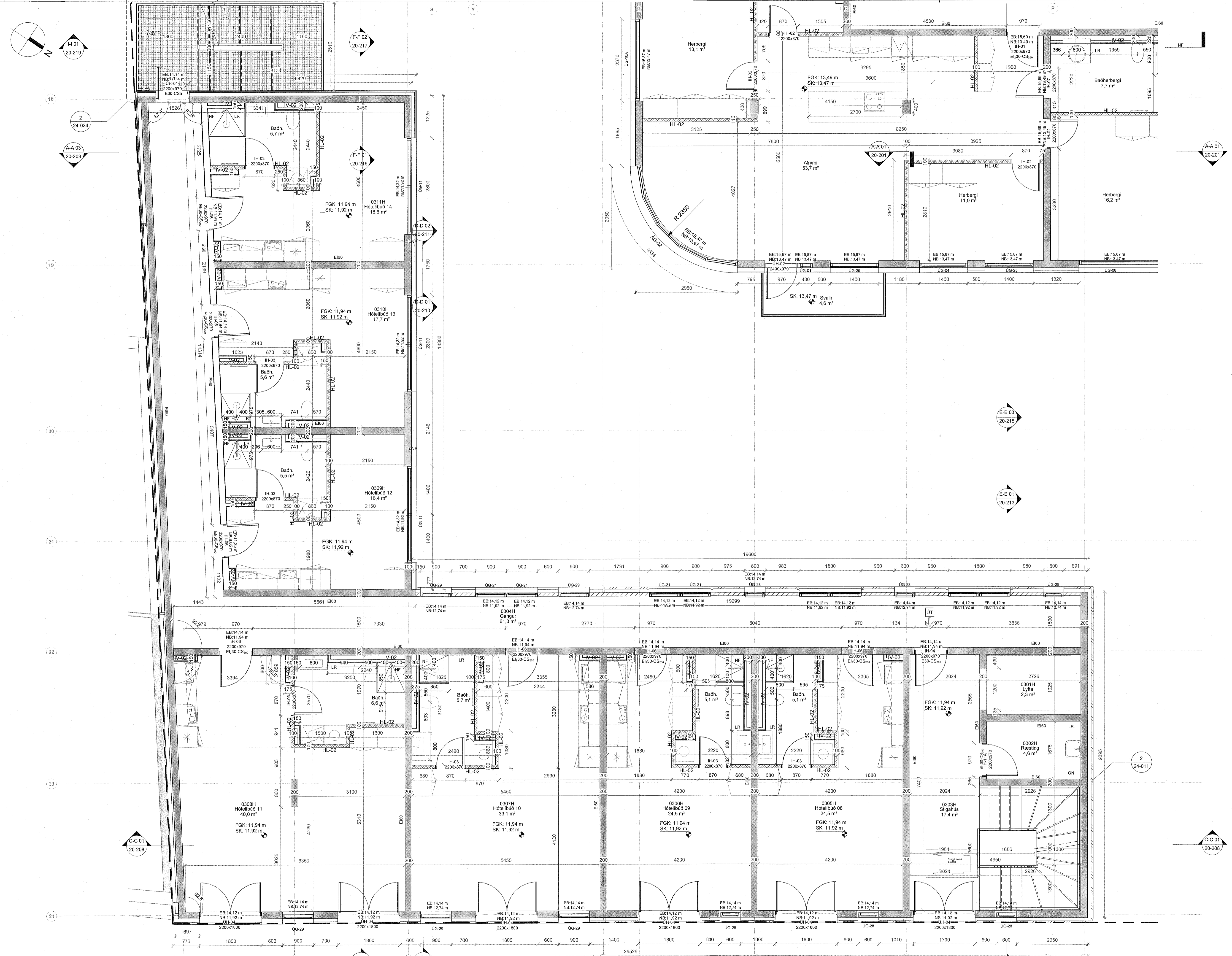
3. hæð Verk. 1-50 - 01 1:50
