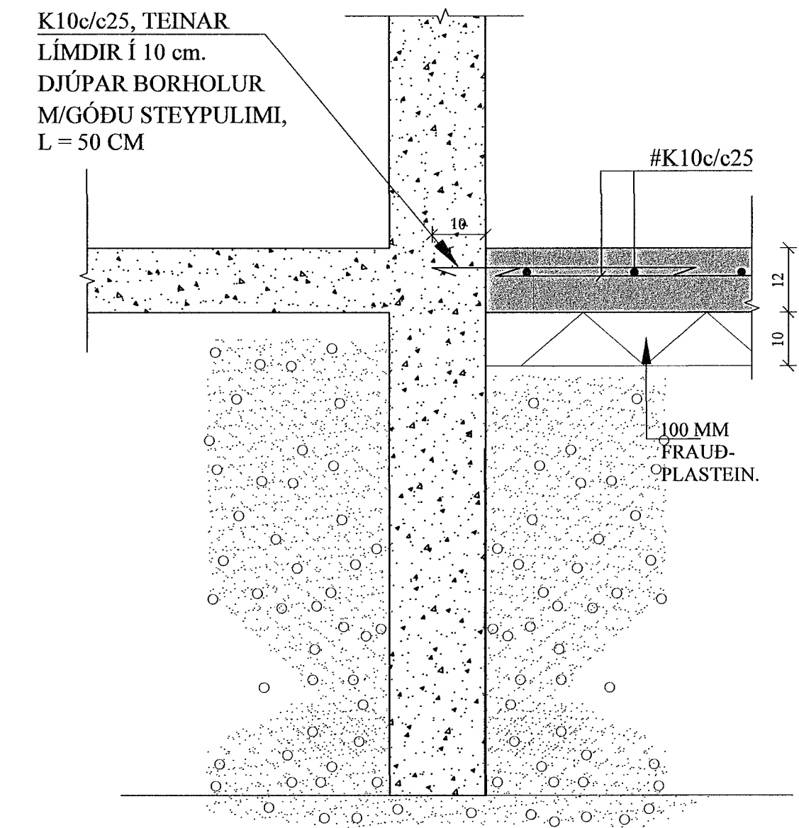
B2 SNIÐ. 1:10 1-02
