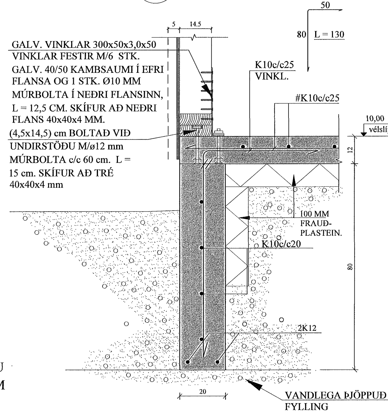
A2 SNIÐ. 1:10 1-02
