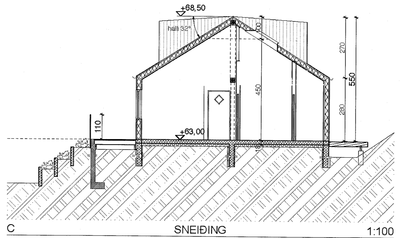
B SNEIÐING 1:100
