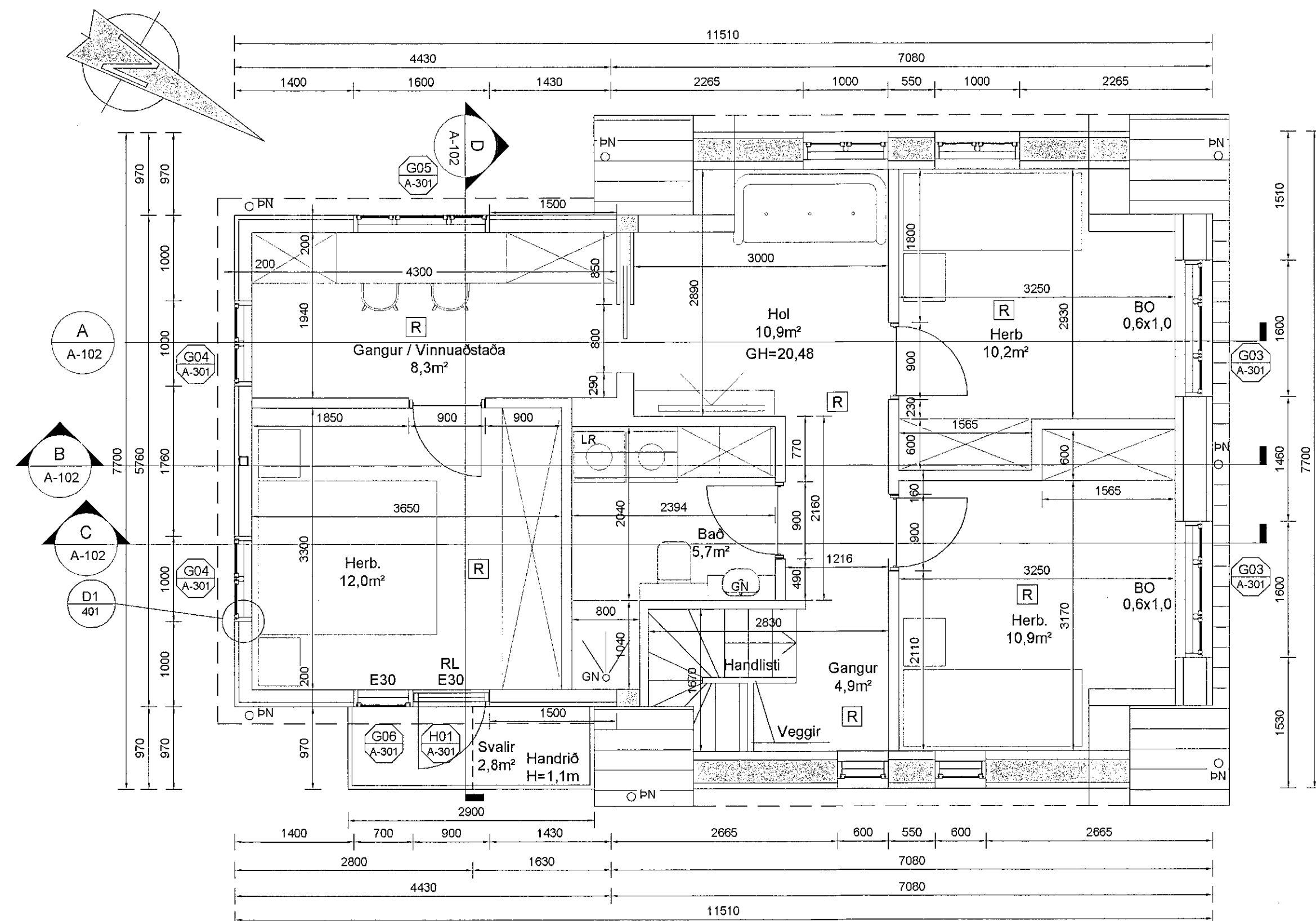
Grunnmynd 2. hæð
