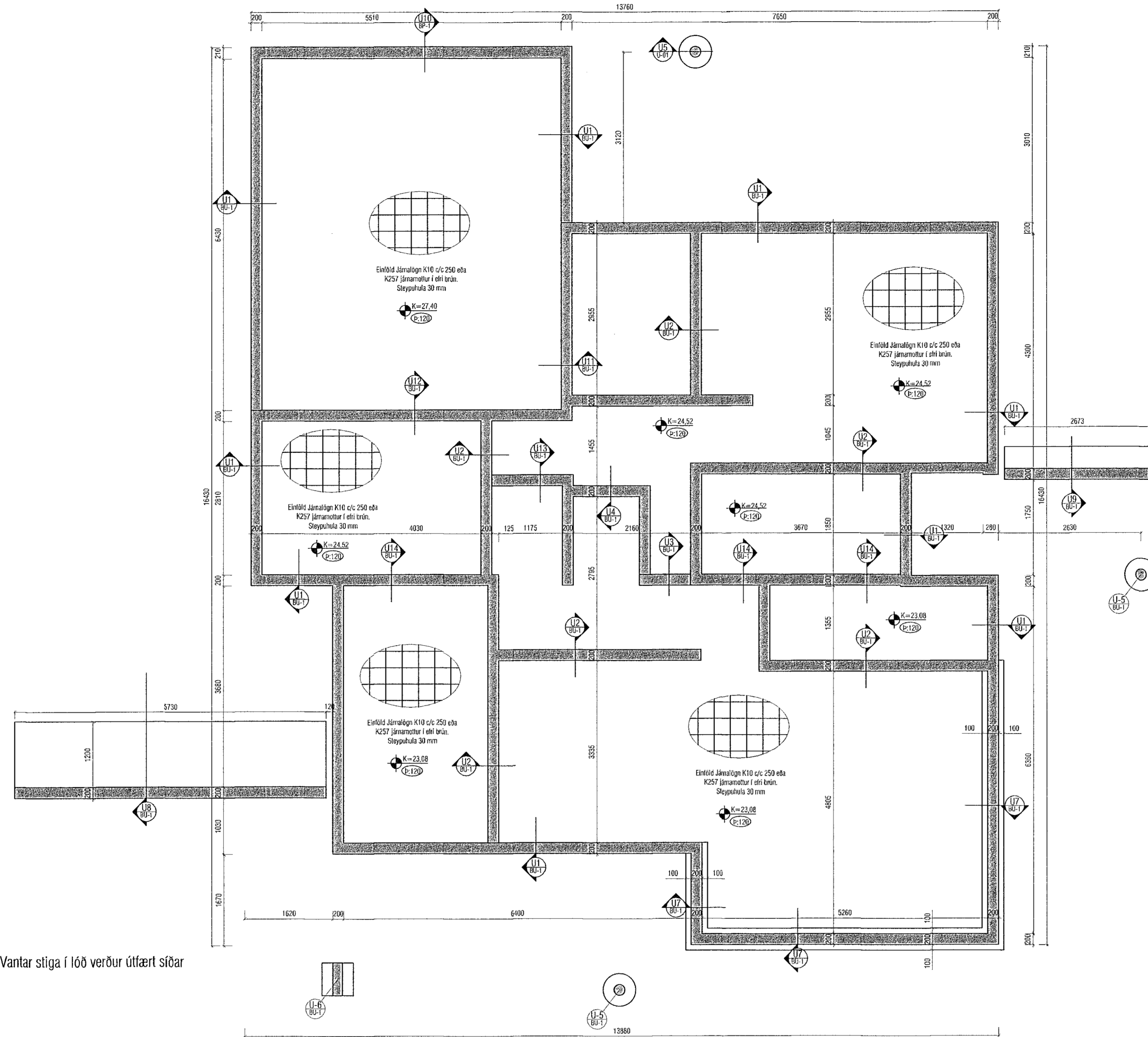
GRUNNMYND UNDIRSTADA MKV. 1:50
