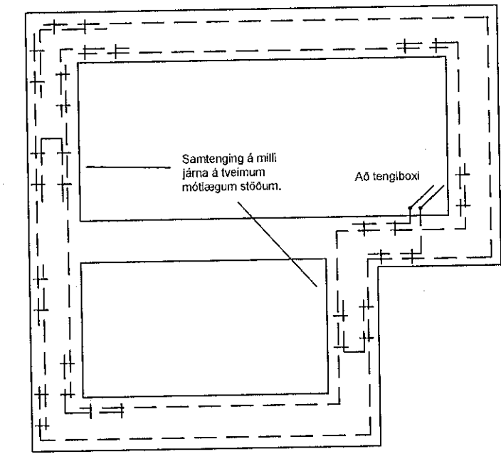
Grundmynd sökkulveggja
