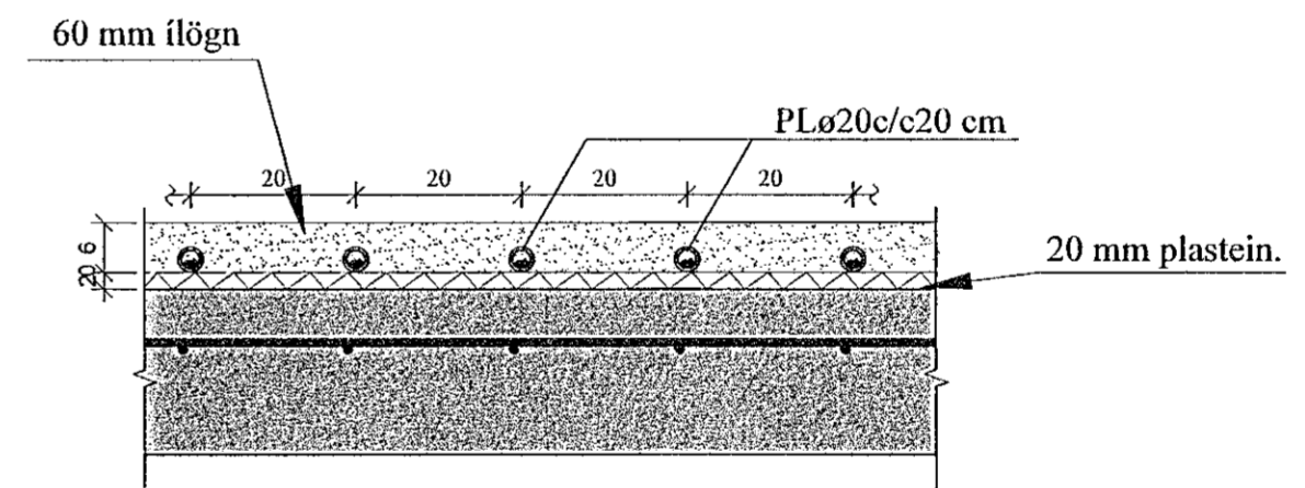
SNIÐ X - X. 1:10 Í SNIÐ X' - X' ER c/c = 20 cm
