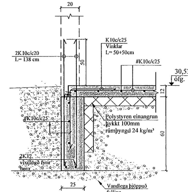
E2 SNIÐ. 1:20 1-02 Útveggur, fyllt að
