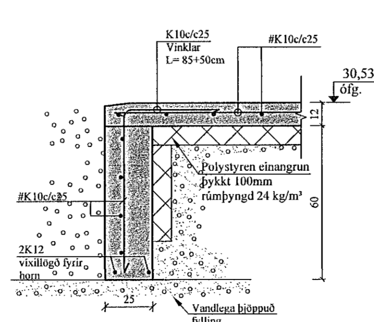
C2 SNIÐ. 1:20 1-02 Útveggur
