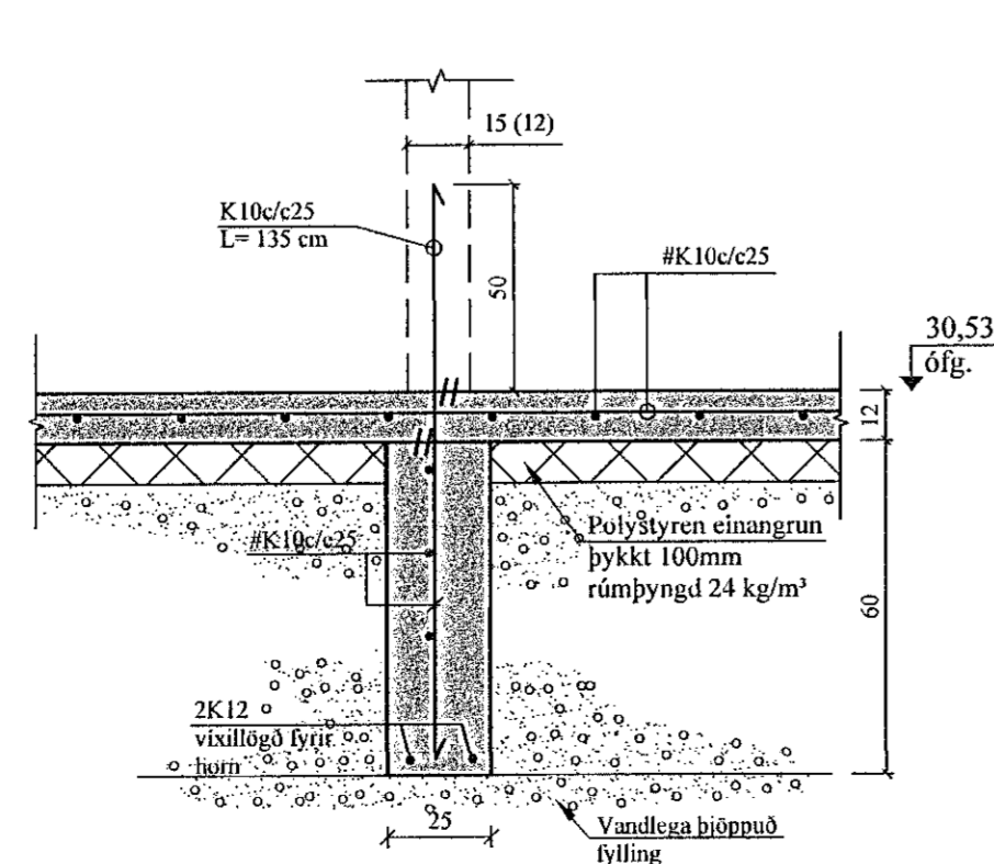
B2 SNIÐ. 1:20 1-02 Innveggur
