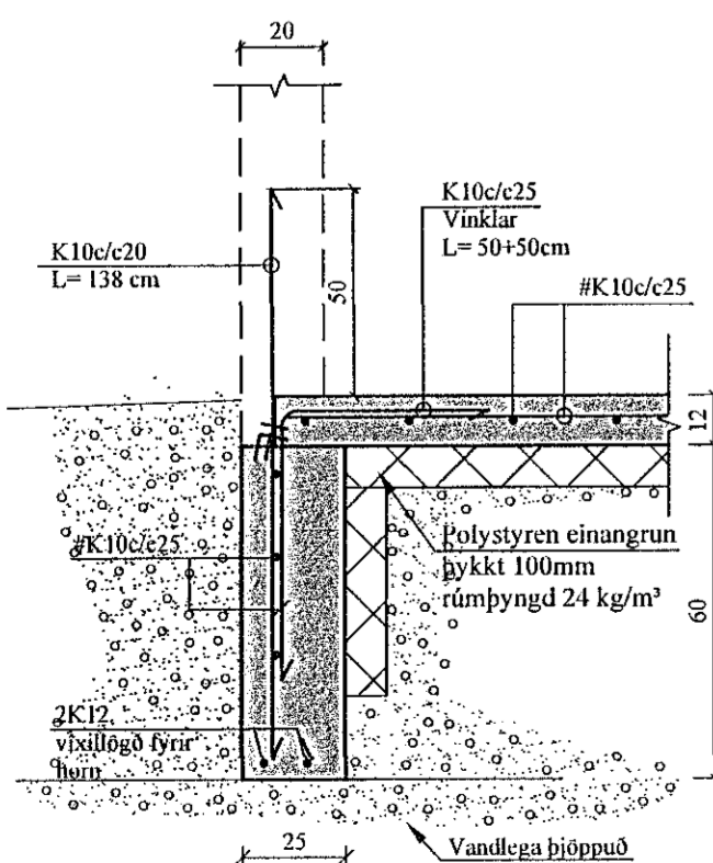
A2 SNIÐ. 1:20 1-02 Útveggur
