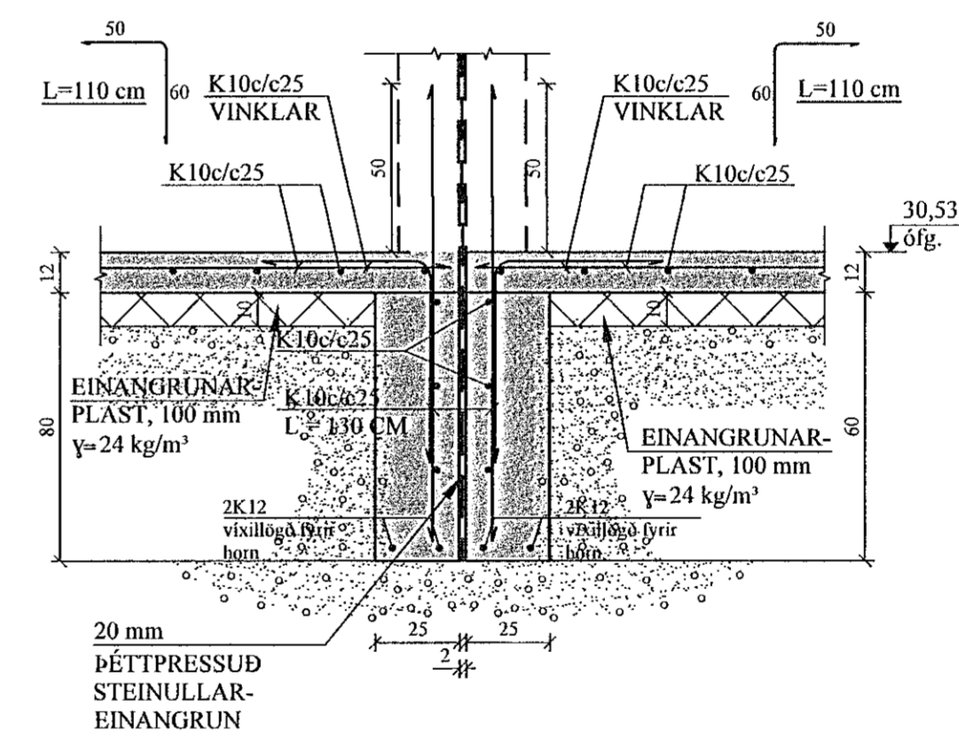
F2 SNIÐ. 1:20 1-02 Milliveggir
