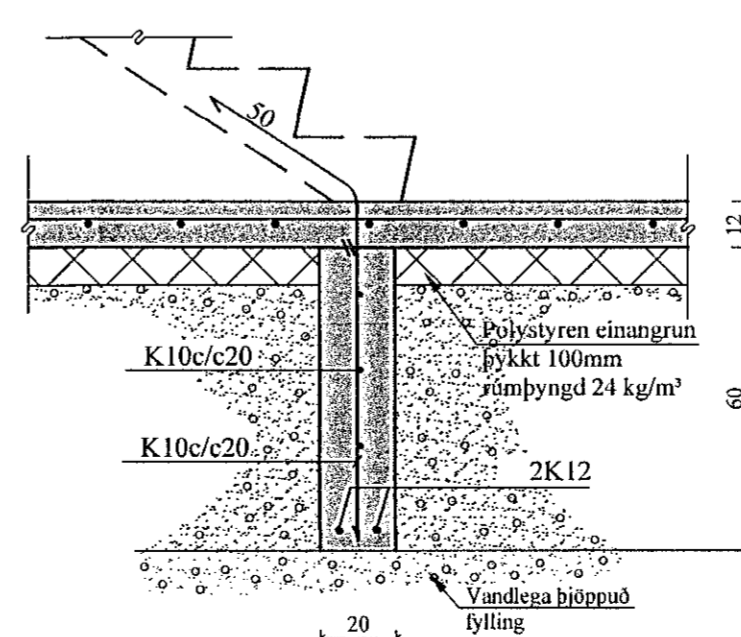
D2 SNIÐ. 1:20 1-02 Stigi
