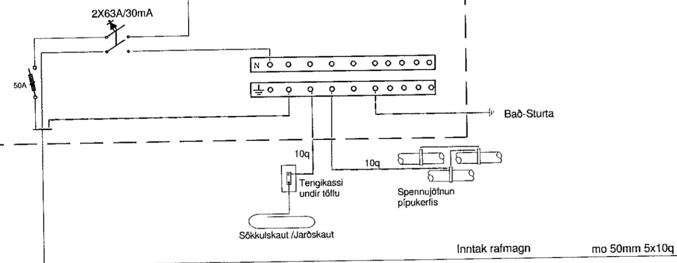
Einlínunmynd greinatafla í íbúð E
