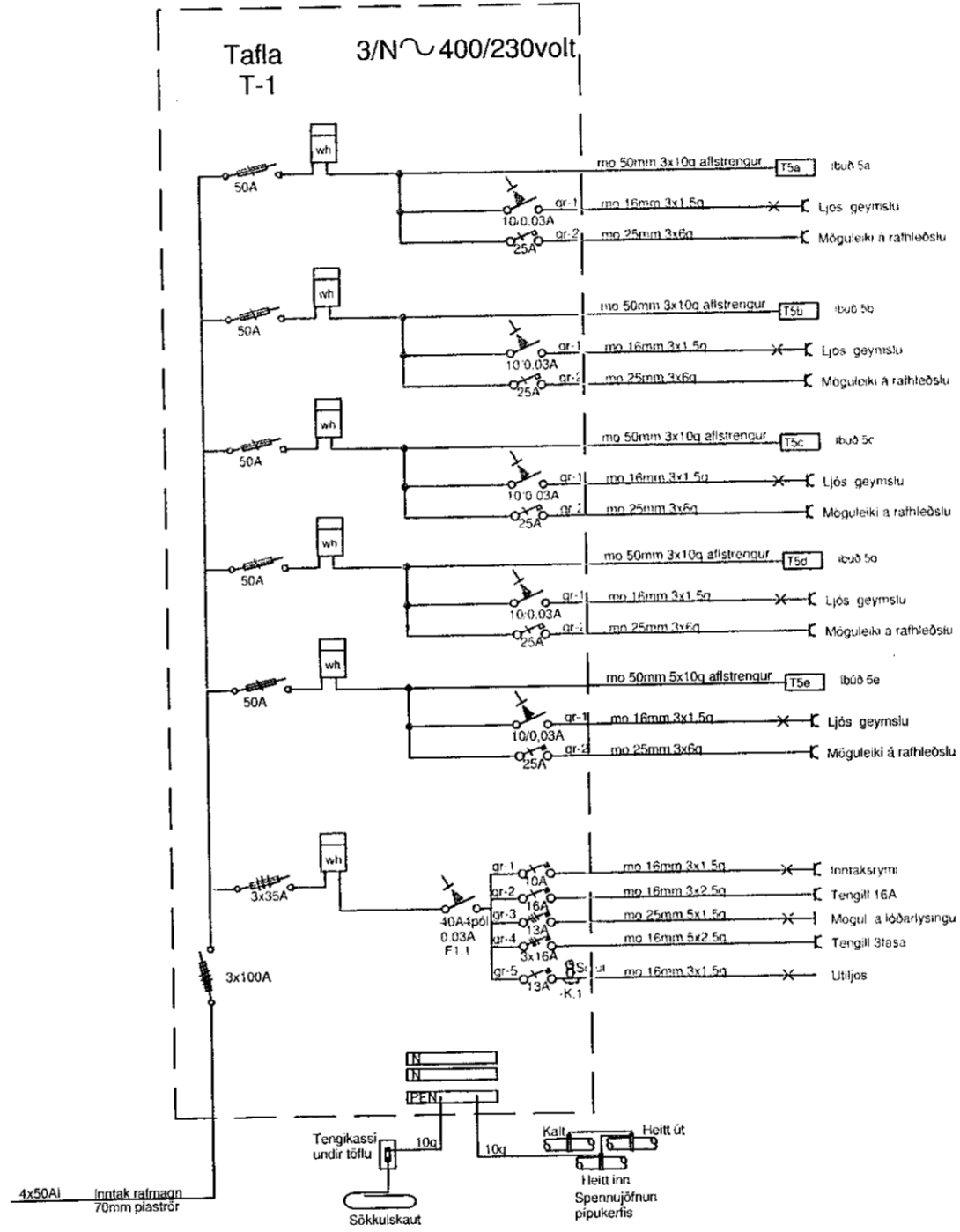
Einlínunmynd Aðaltafla í innt.rymi
