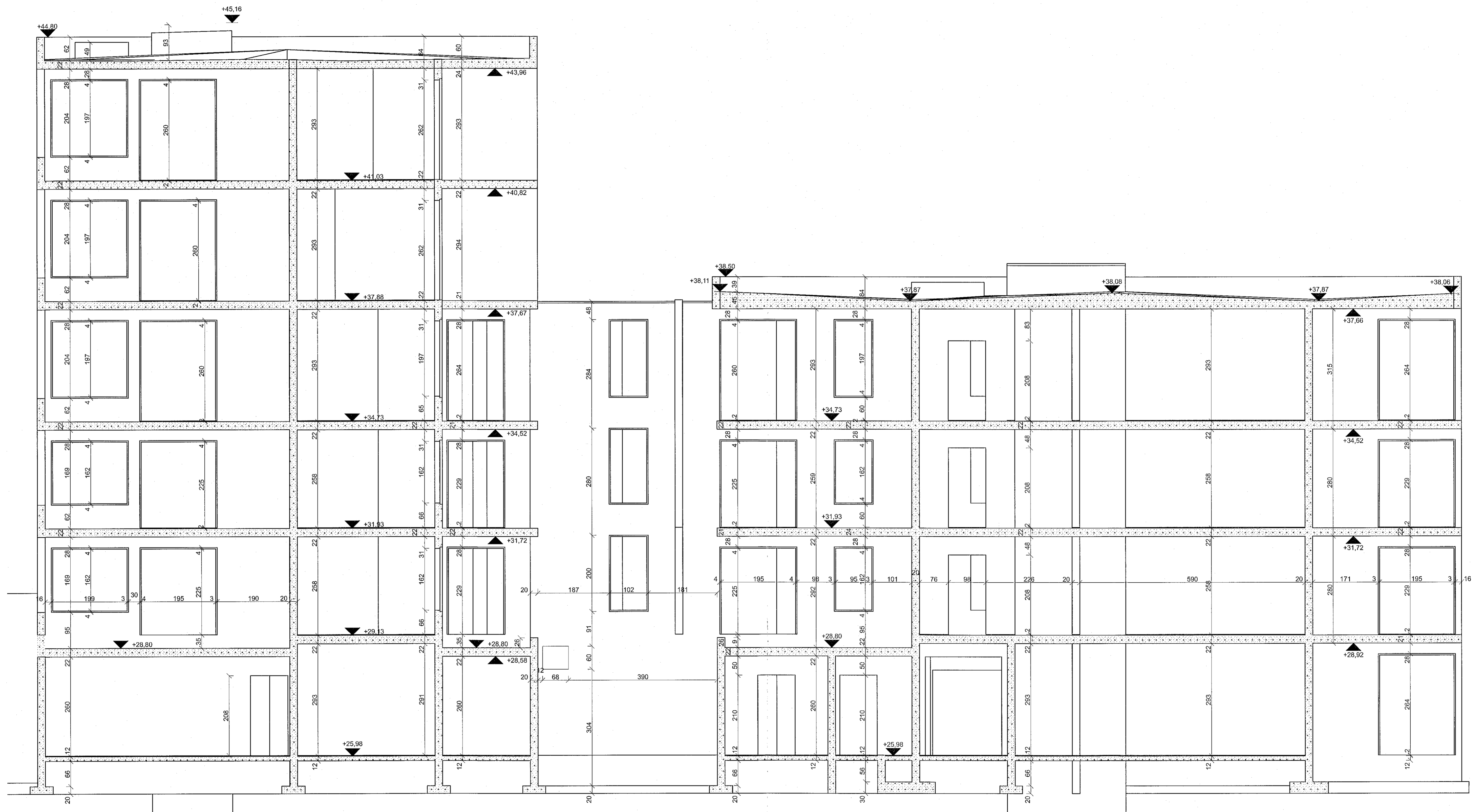
A-05 Svalir 1:50
