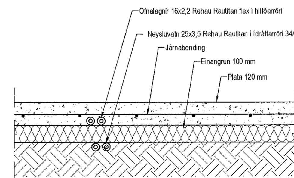
Hita- og vatnslagnir, Sníð í botnplötu, 1:10
