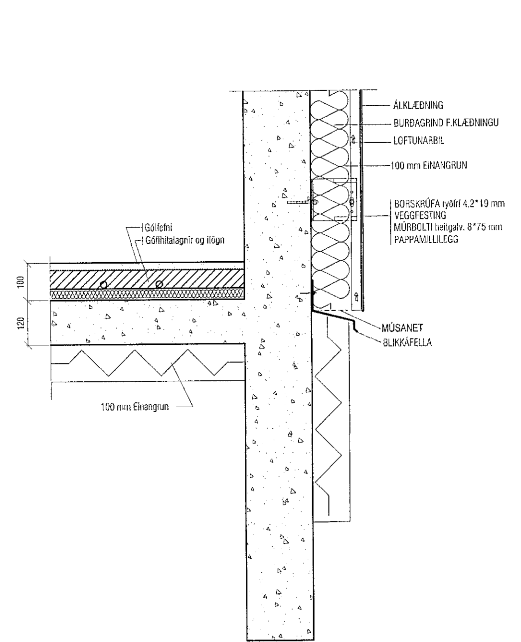
1:10 DEILI 4 S-09/10
