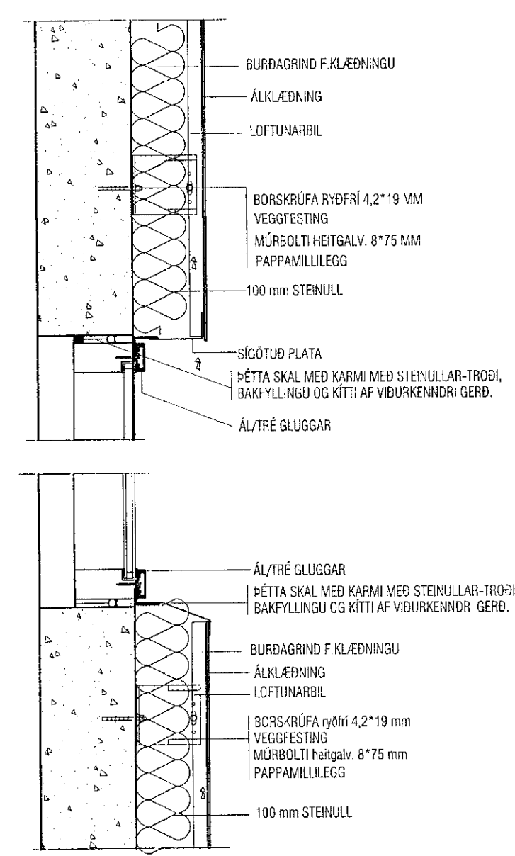
1:10 DEILI 3 S-09/10
