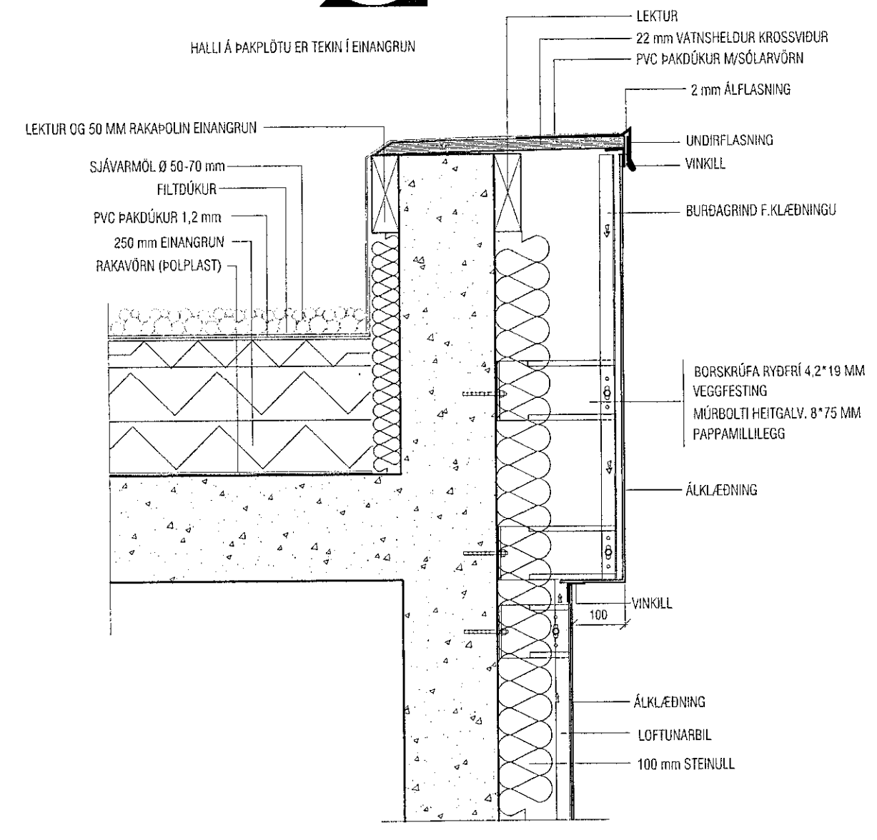
1:10 DEILI 4 S-09/10
