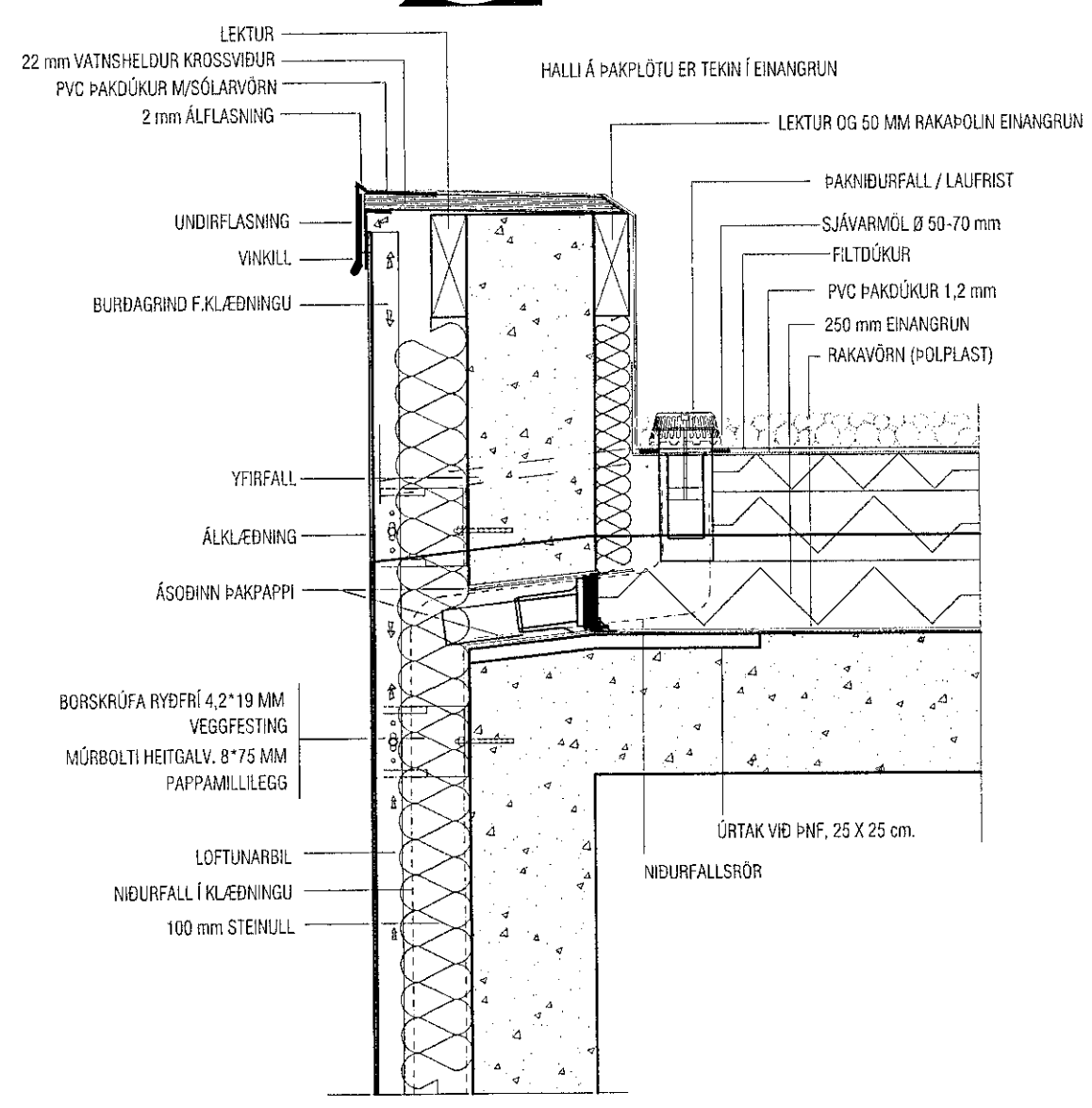
1:10 DEILI 3 S-09/10
